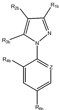
(IB)
