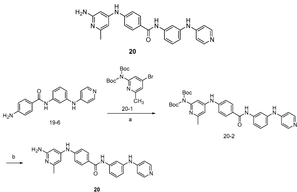
반응식 15
