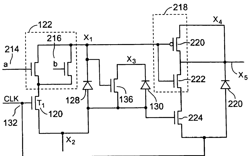
FIG. 7C OR-2 GATE
