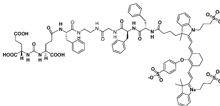
PET agent conjugate
