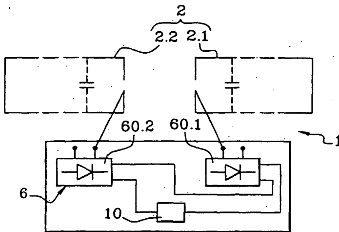
Fig. 7D
