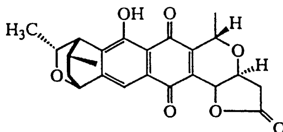
GRANATICIN (4)
