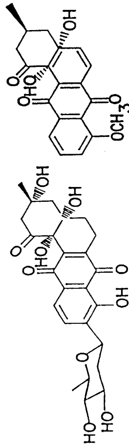
RUBIGINONE A 2
