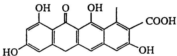
TETRACENOMYCIN F1 (5)
