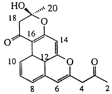
RM 20 (9)
