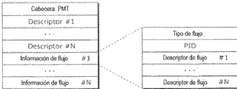
Estructura de datos de la PMT
