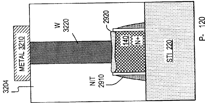
FIG. 25C (PERIPHERY)
