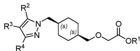
(1 s ,4 s )- or cis - mesoisomer
