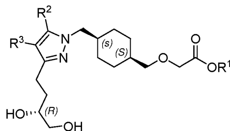
(1 S ,4 s )- or cis -
