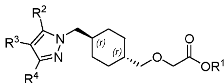
(1 r ,4 r )- or trans - mesoisomer
