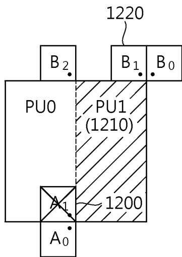
Nx2N
