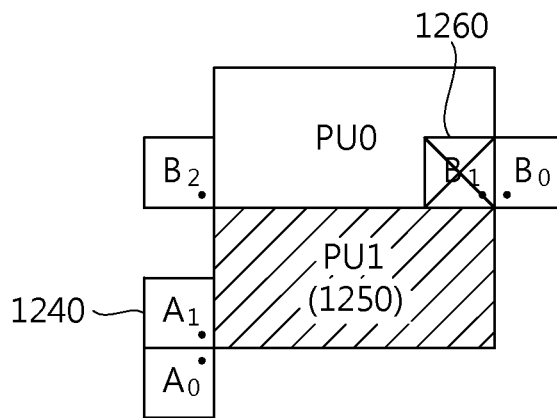
2NxN
