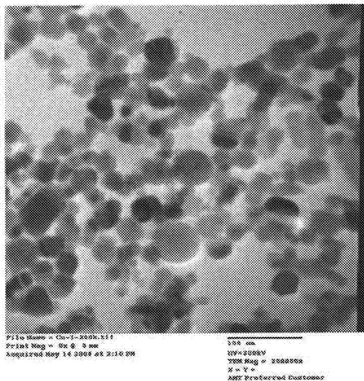
FIG. 5 TEM Copper II-Oxide
