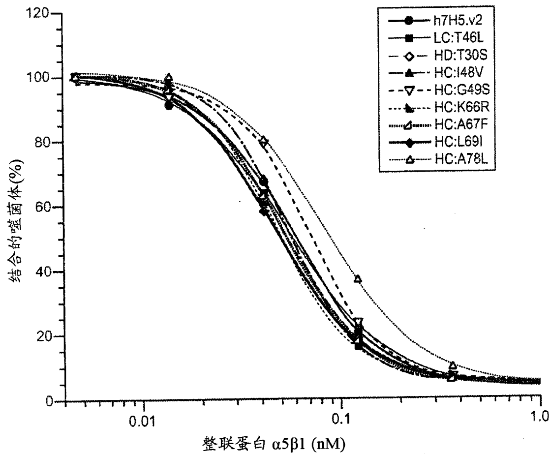
h7H5.v2 框架变体的噬菌体竞争 ELISA
