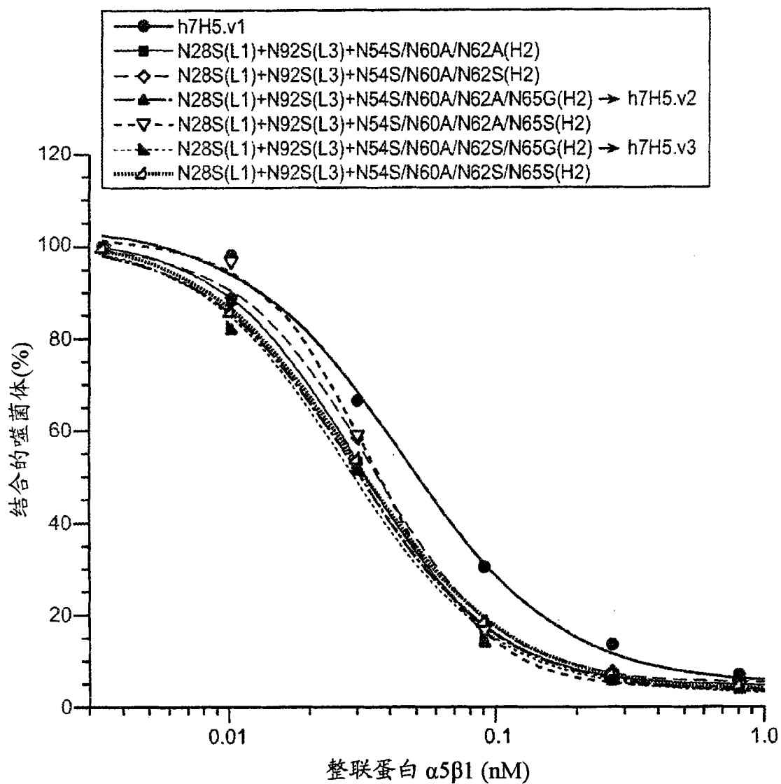
h7H5.v1 CDR 多点突变体的噬菌体竞争 ELISA
