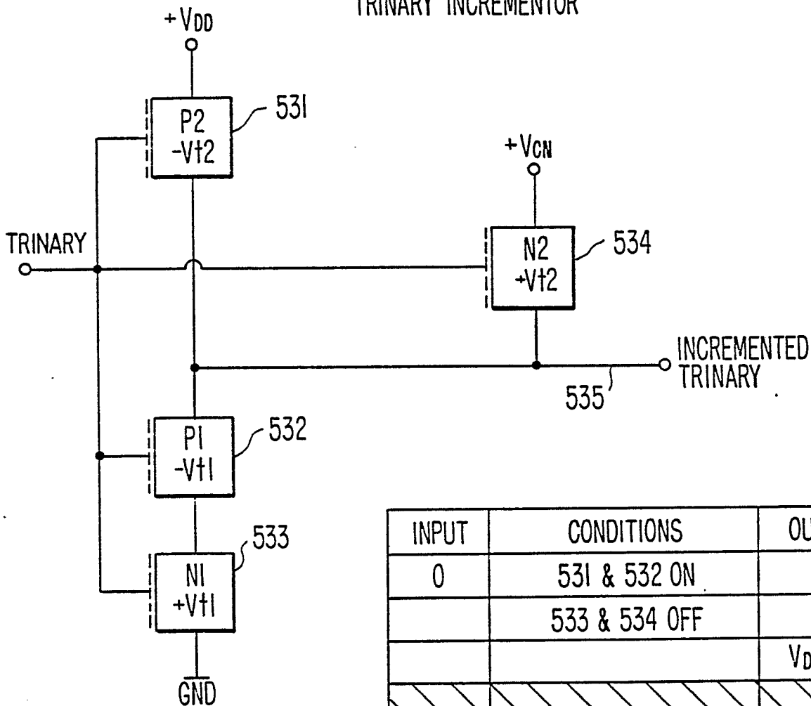
FIG. 14A. TRINARY INCREMENTOR
