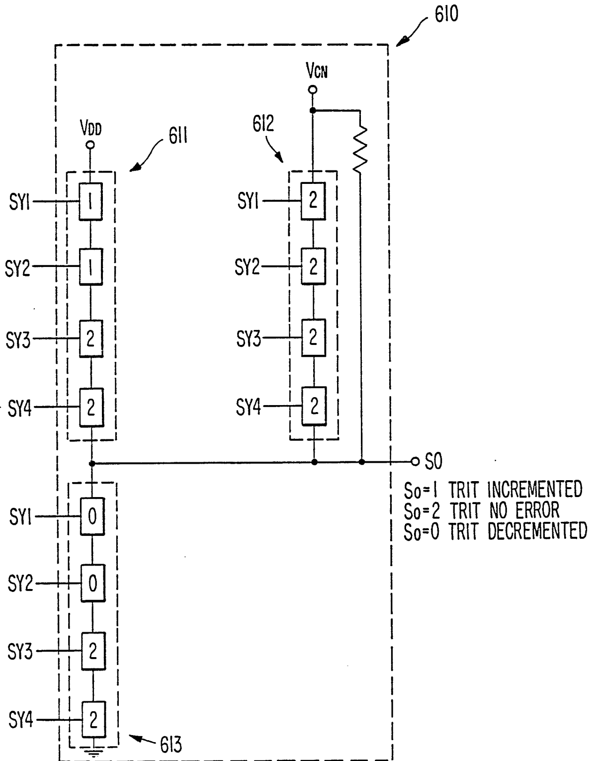
FIG. 11A. SINGLE ERROR DETECTOR
