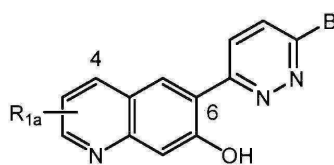
(Ia8)
