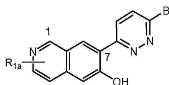
(Ia9)
