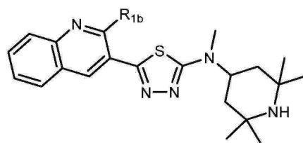
(화학식 Ib8)
