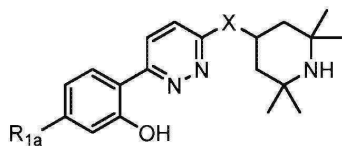
(Ia15)
