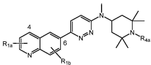
(Ia2)
