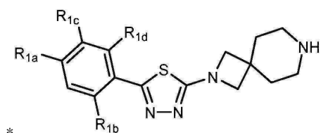
(Ib6)
