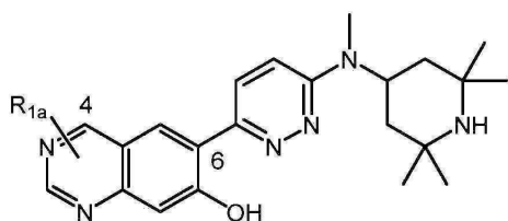
(Ia7)
