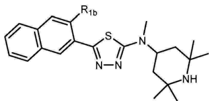
(Ib7)
