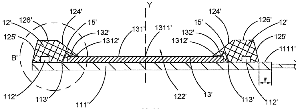
A'-A' FIG. 33
