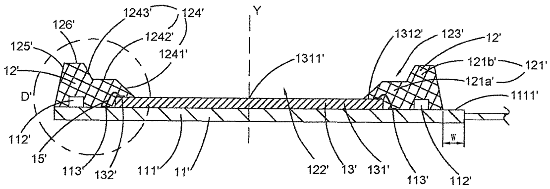
C'-C' FIG. 42
