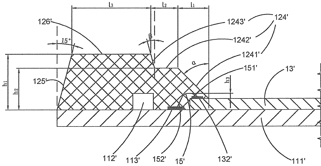
FIG.59
