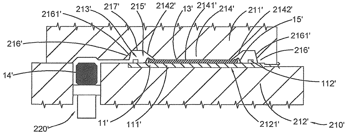
A'-A' FIG.36A
