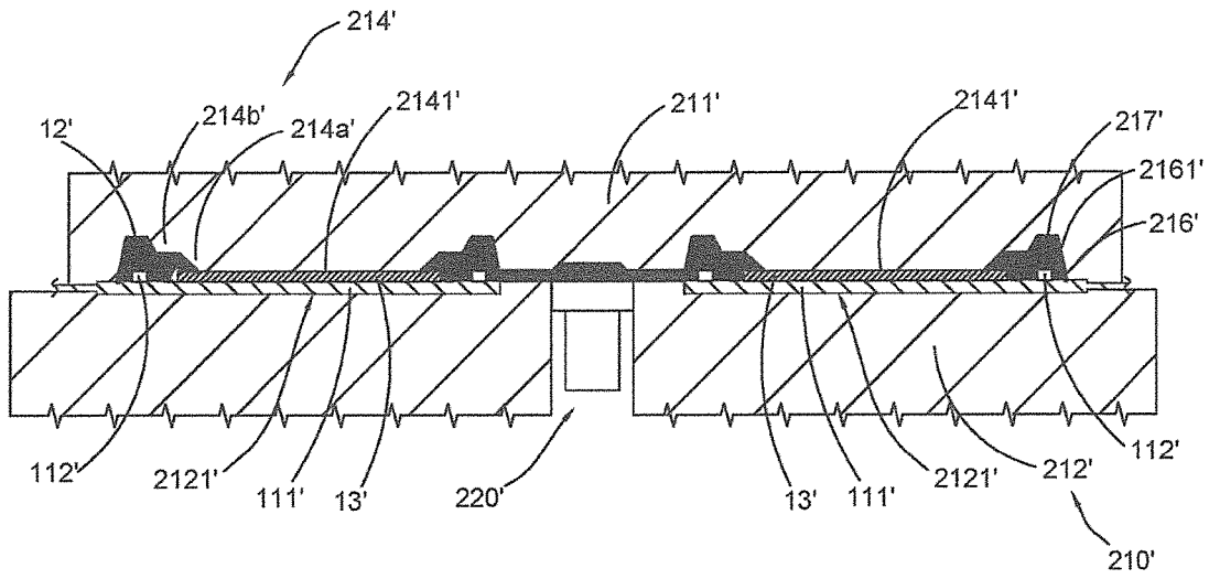
C'-C' FIG. 45
