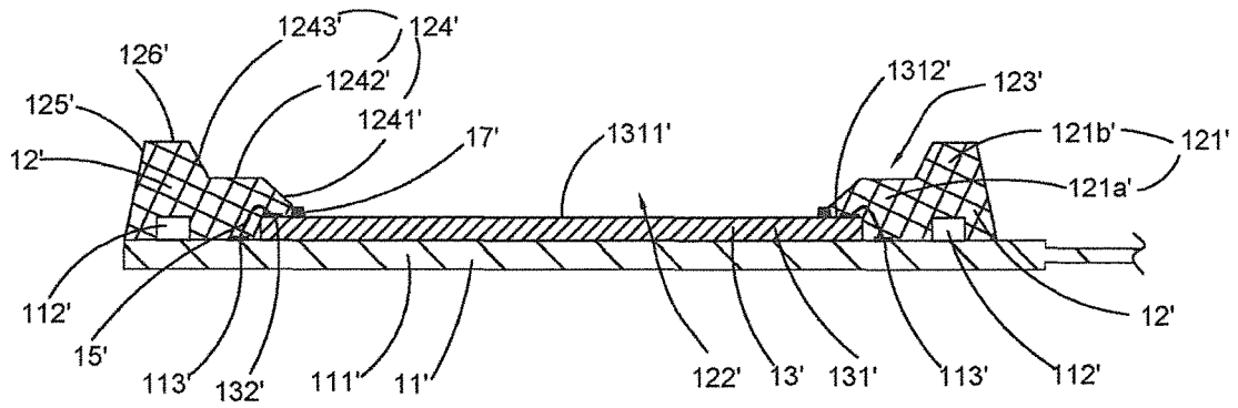
FIG. 52
