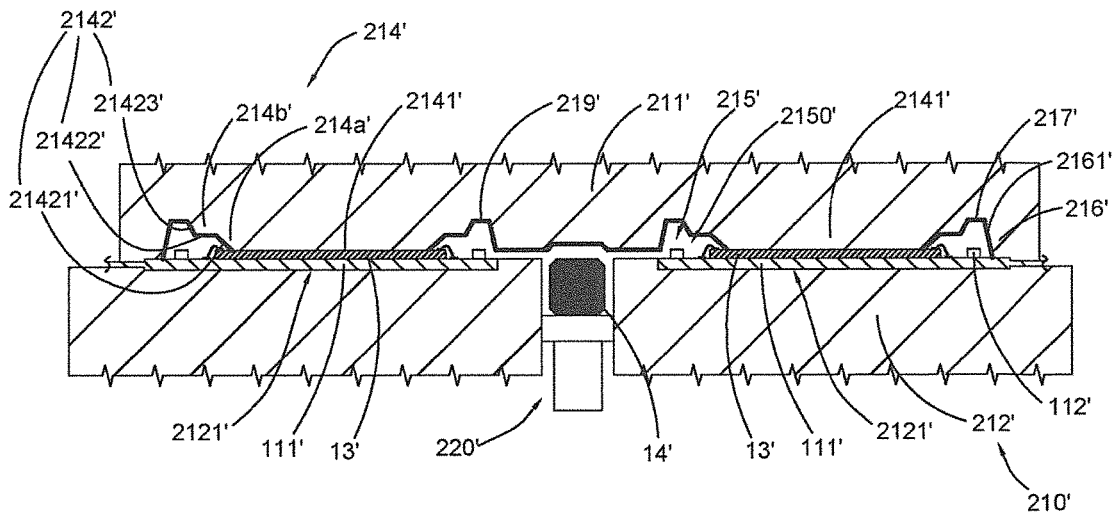
FIG. 44
