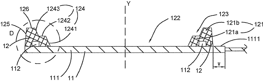
C-C FIG 14
