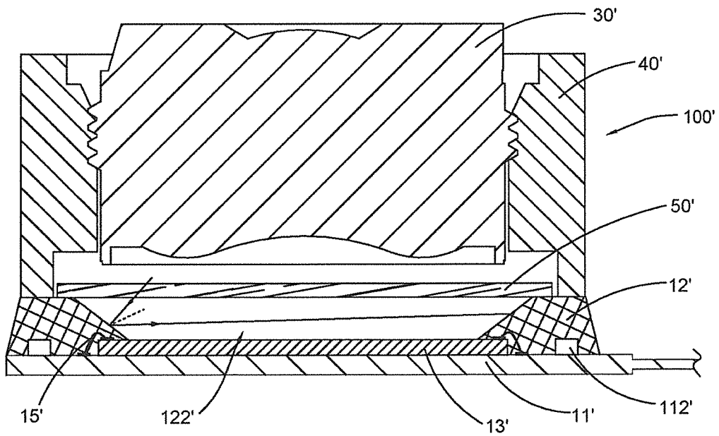
FIG. 35
