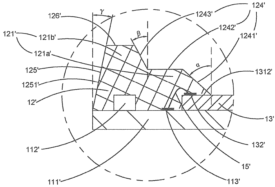
D' FIG. 43
