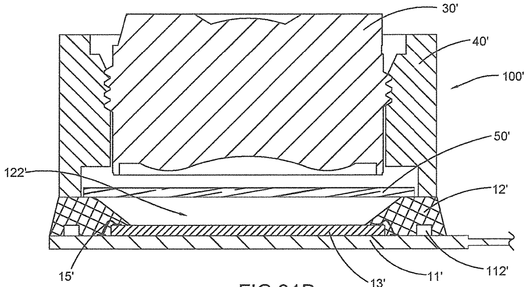
FIG. 31B
