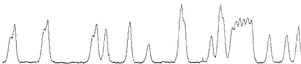
DTAMRA-2-labeled ddCTP using a propargyl-1-ethoxyamido linker
