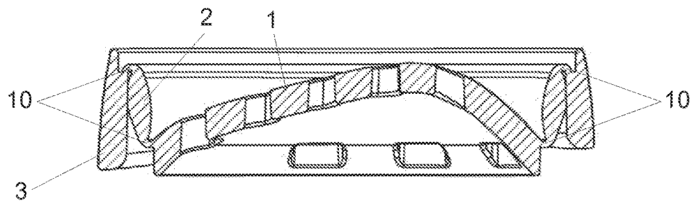
C - C FIG. 9b
