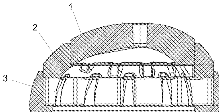
A - A FIG. 4a
