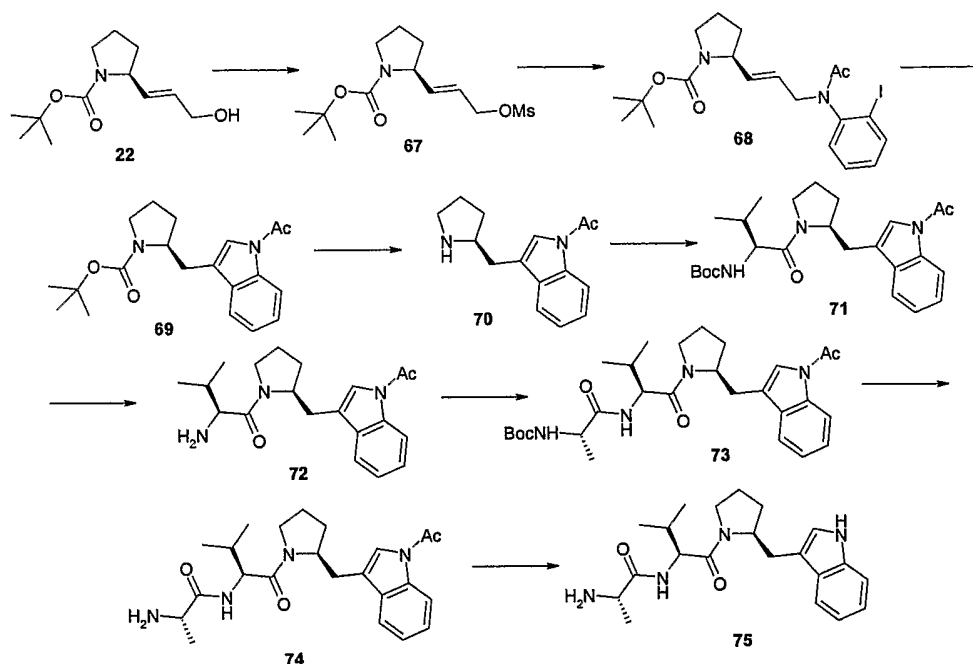
Scheme VI
