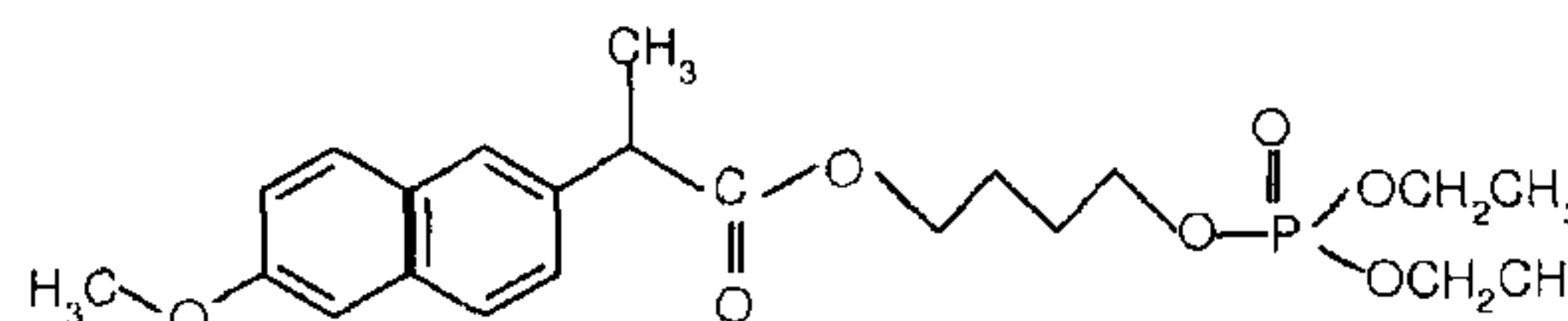
Phospho-naproxen
