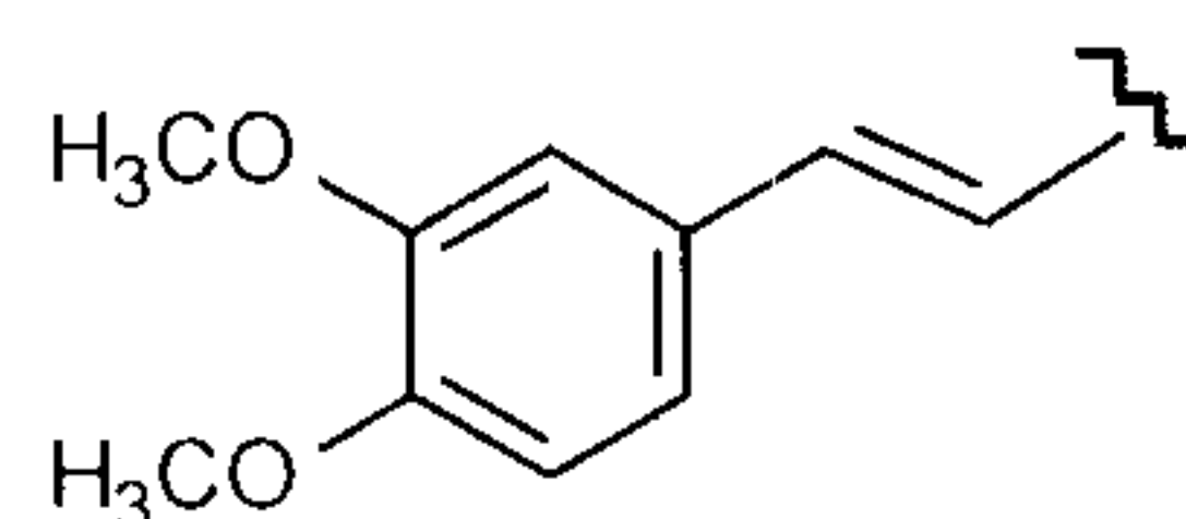
Formula (VIIb)
