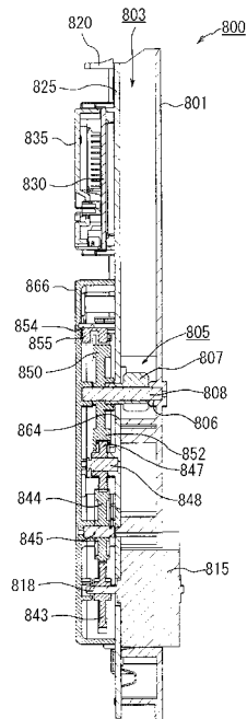
A-A 断面図
