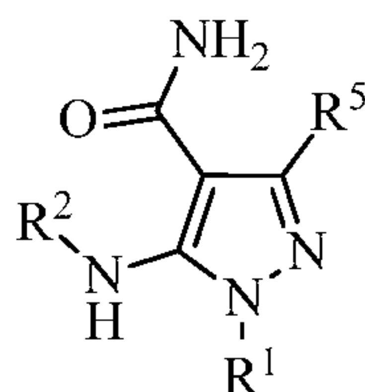
(III-b)
