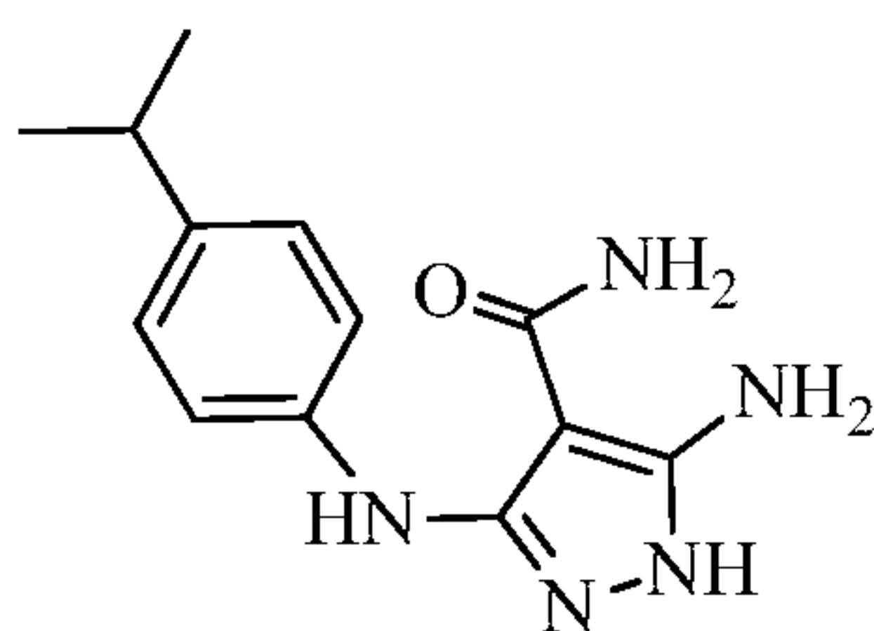
5-amino-3-((4-isopropylphenyl)amino)-1 H -pyrazole-4-carboxamide
