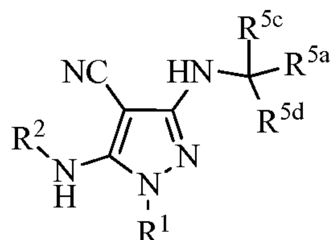
(XIV-b)
