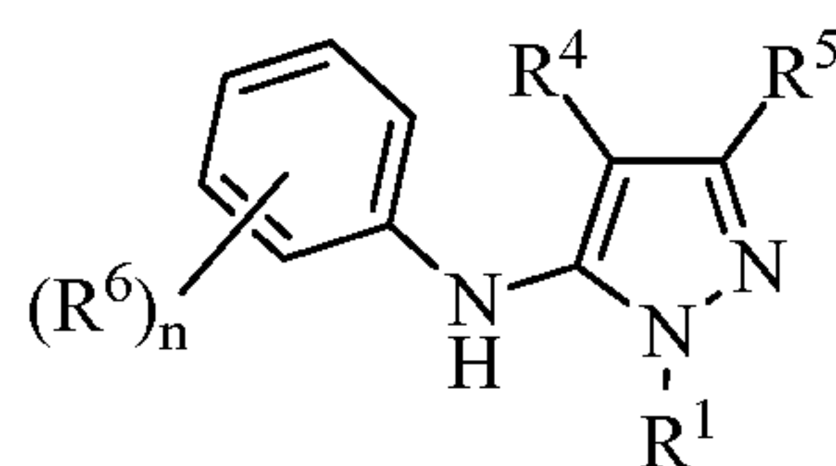
(IV-b)
