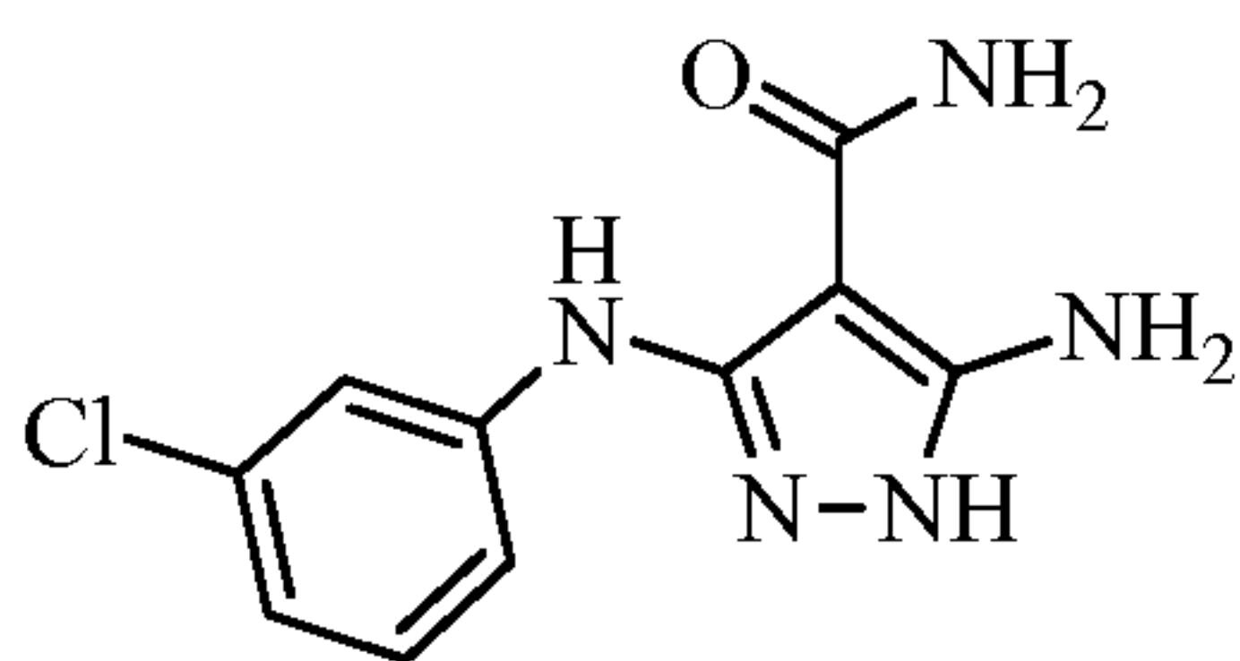
5-amino-3-((3-chlorophenyl)amino)-1 H -pyrazole-4-carboxamide
