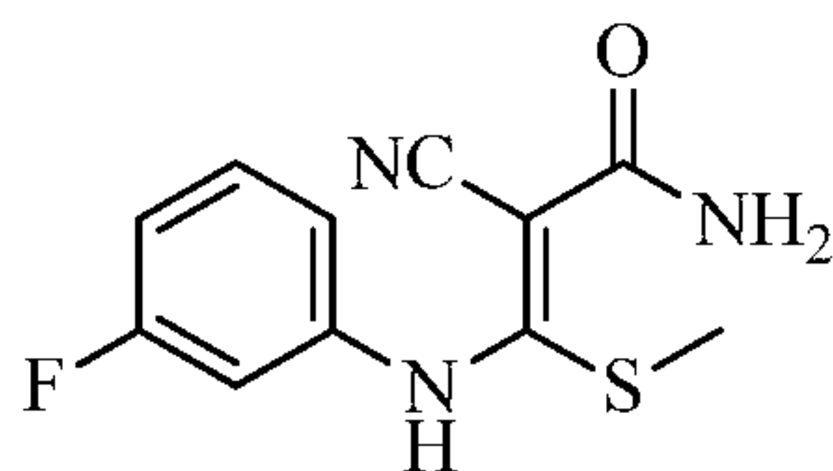
2-cyano-3-((3-fluorophenyl)amino)-3-(methylthio)acrylamide
