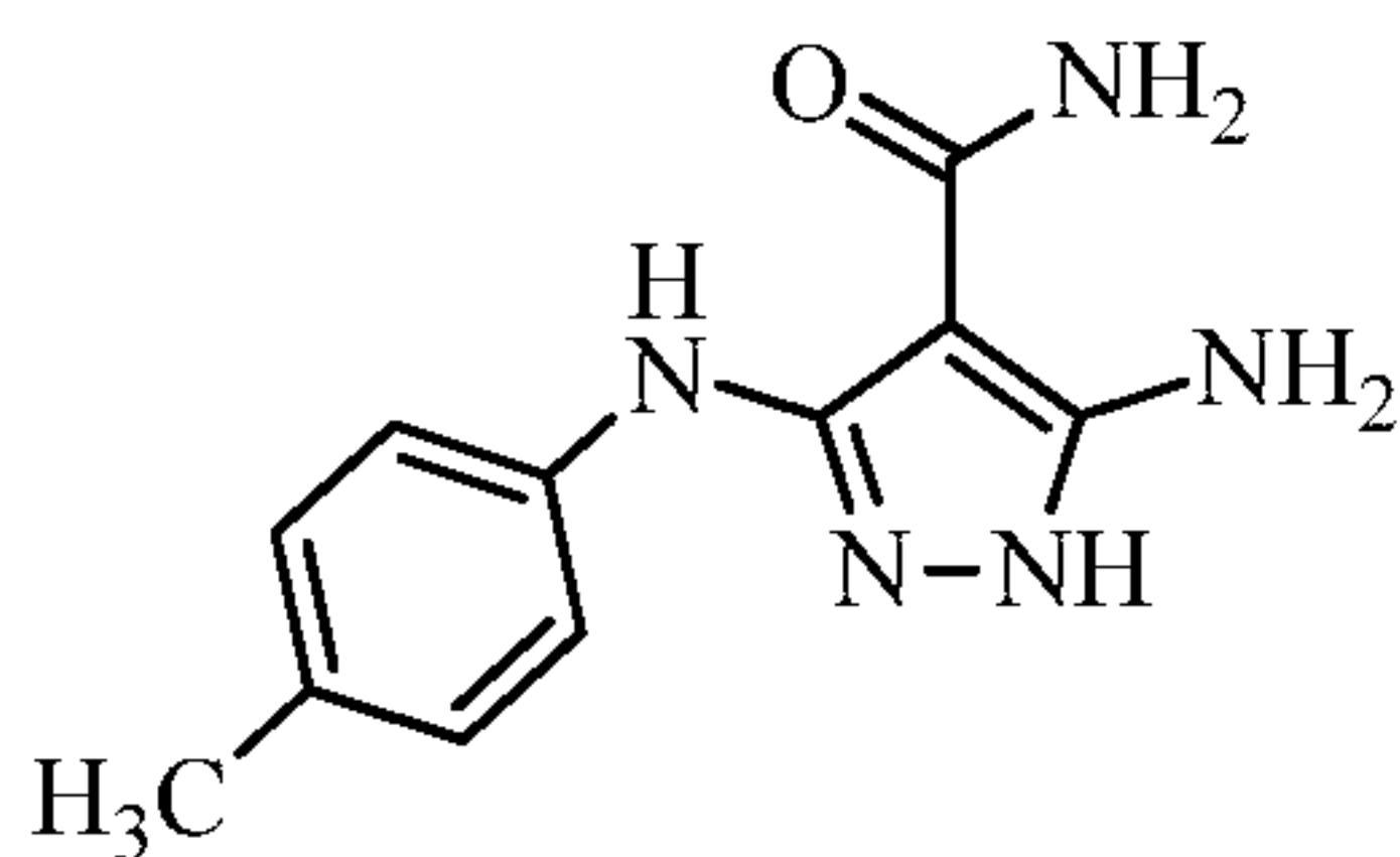
5-amino-3-( p -tolylamino)-1 H -pyrazole-4-carboxamide
