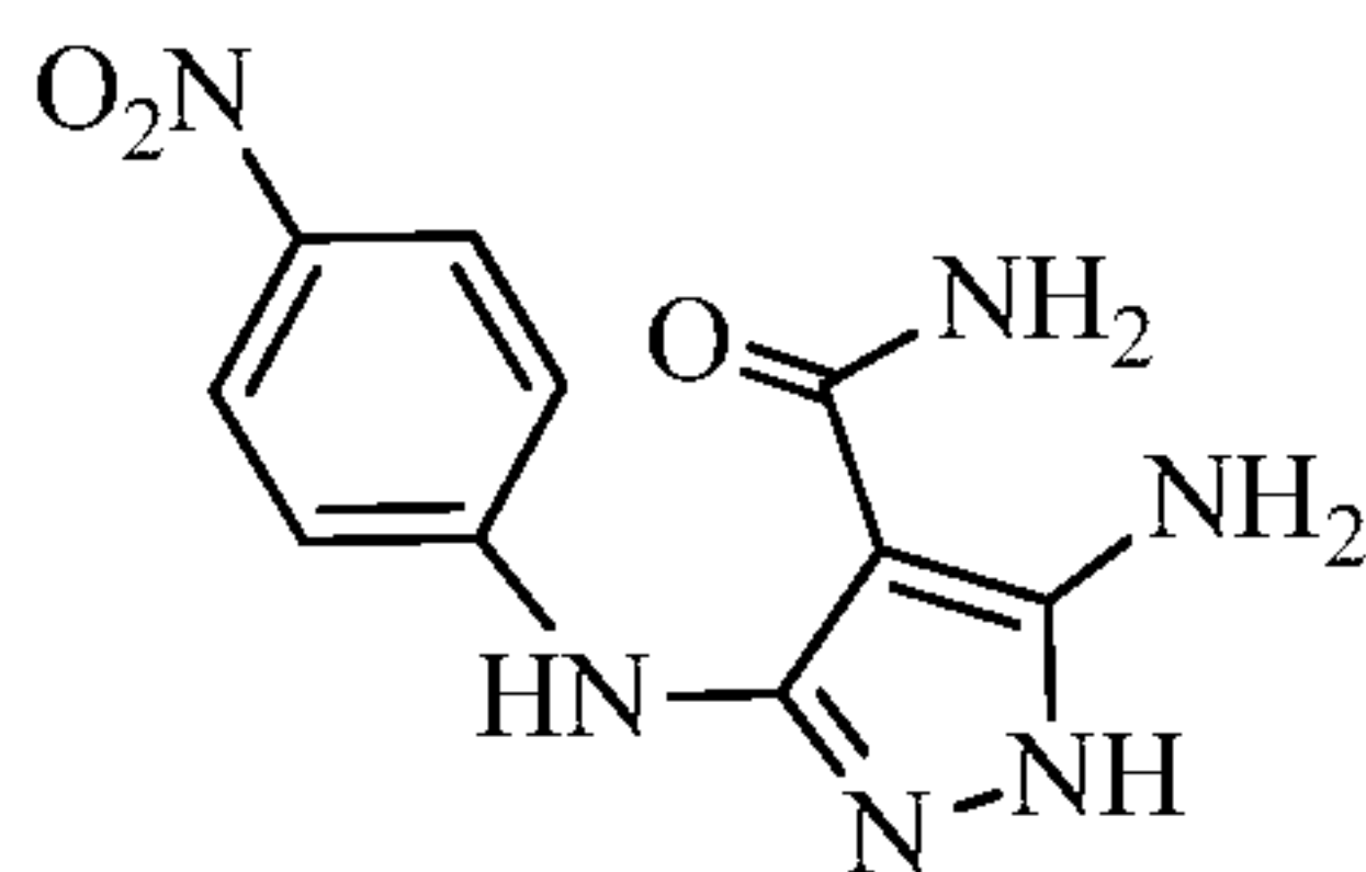
5-amino-3-((4-nitrophenyl)amino)-1 H -pyrazole-4-carboxamide
