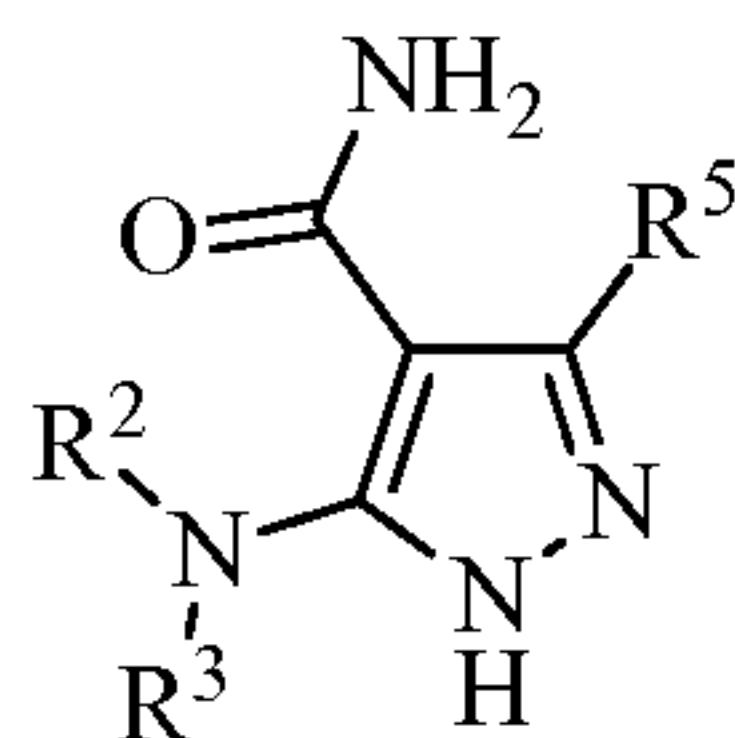
(III-a)
