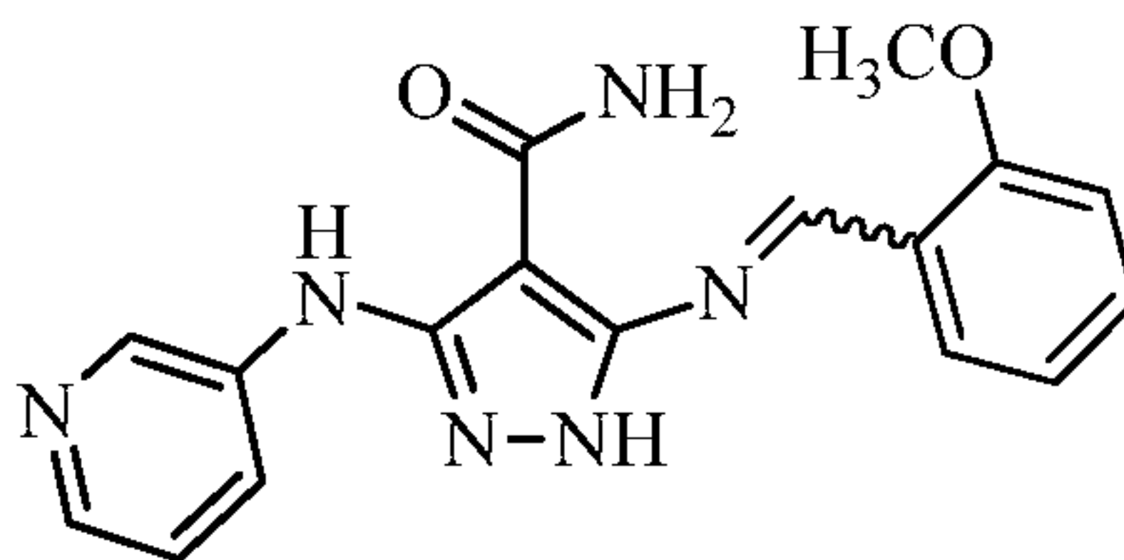
5-((2-methoxybenzylidene)amino)-3-(pyridin-3-ylamino)-1 H -pyrazole-4-carboxamide
