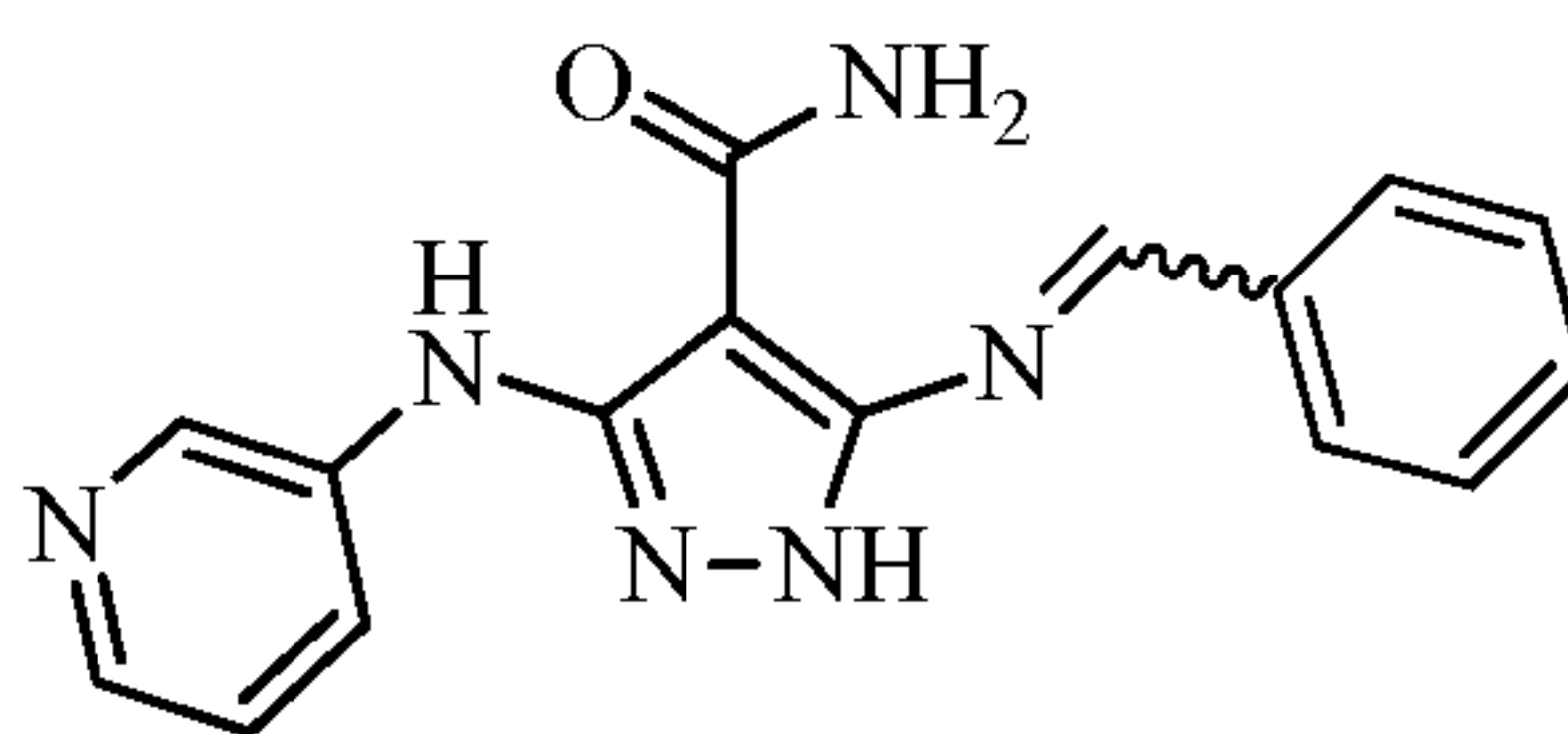
5-(benzylideneamino)-3-(pyridin-3-ylamino)-1 H -pyrazole-4-carboxamide
