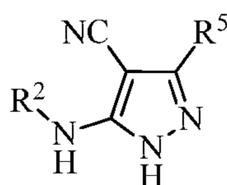
(II-c)
