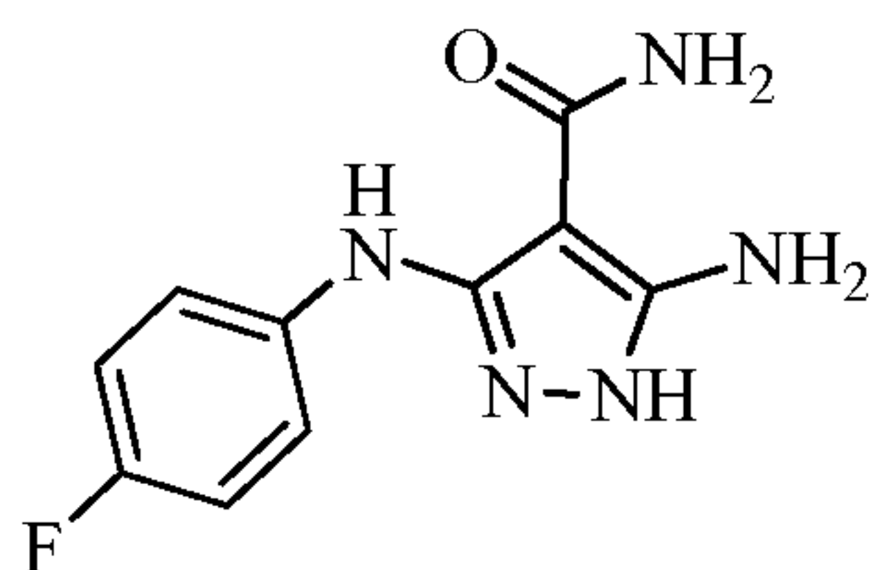
5-amino-3-((4-fluorophenyl)amino)-1 H -pyrazole-4-carboxamide
