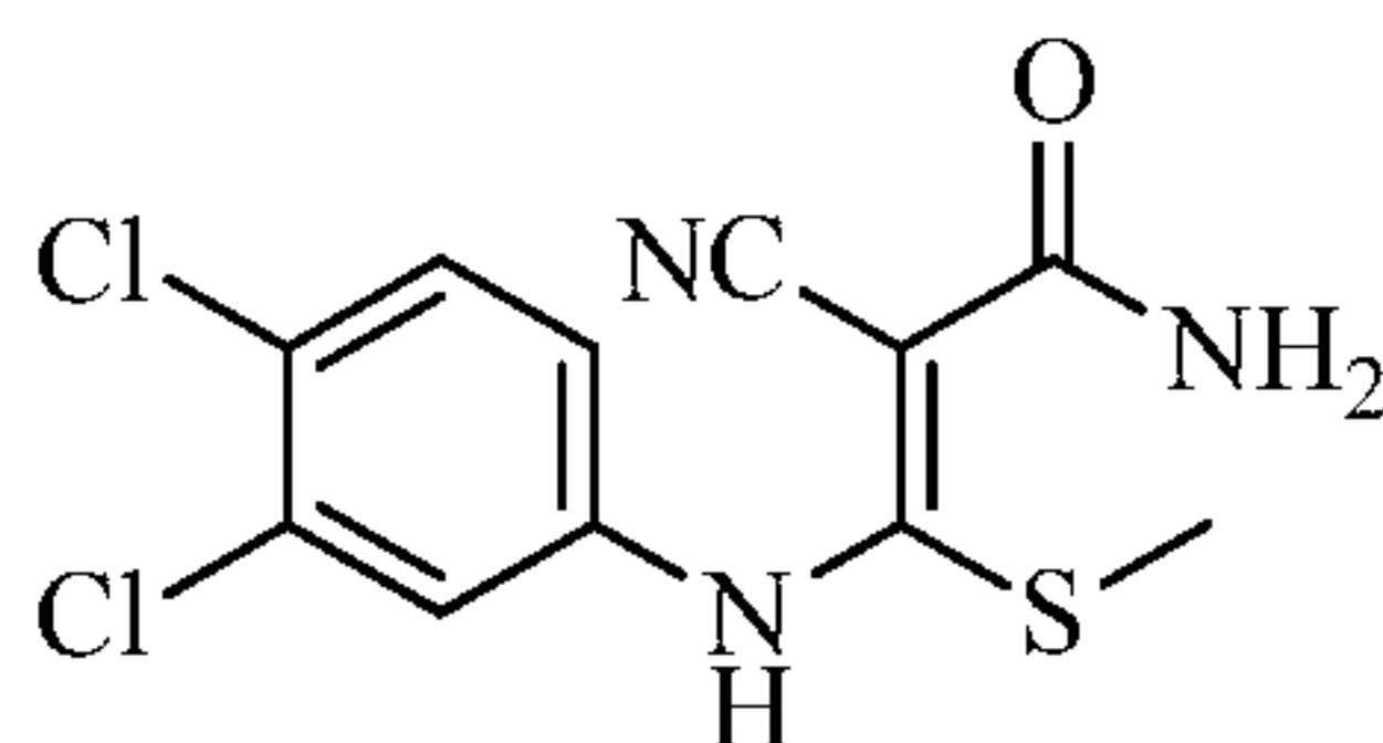
2-cyano-3-((3,4-dichlorophenyl)amino)-3-(methylthio)acrylamide
