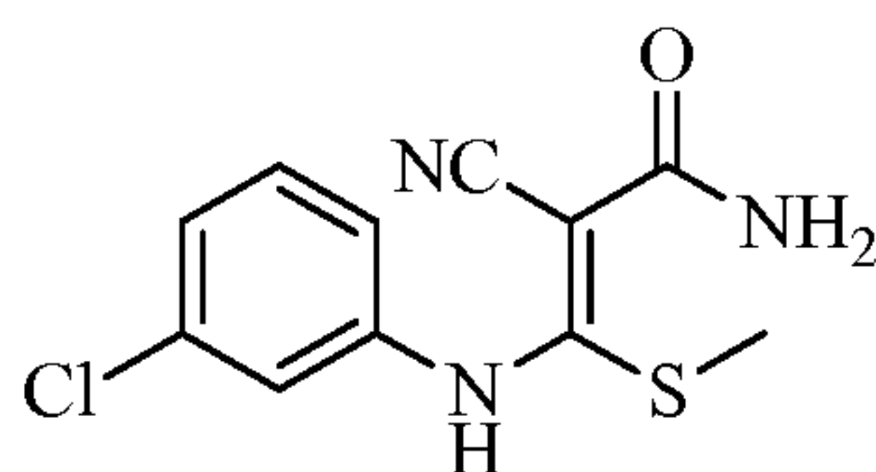
3-((3-chlorophenyl)amino)-2-cyano-3-(methylthio)acrylamide
