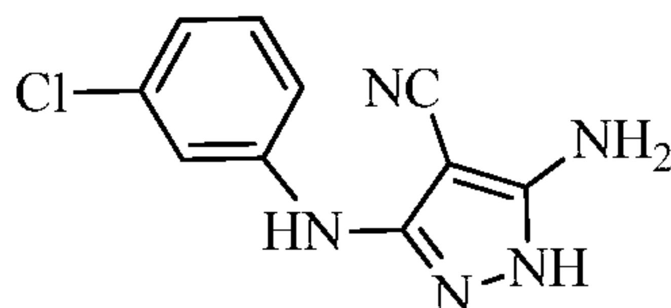
5-amino-3-((3-chlorophenyl)amino)-1 H -pyrazole-4-carbonitrile
