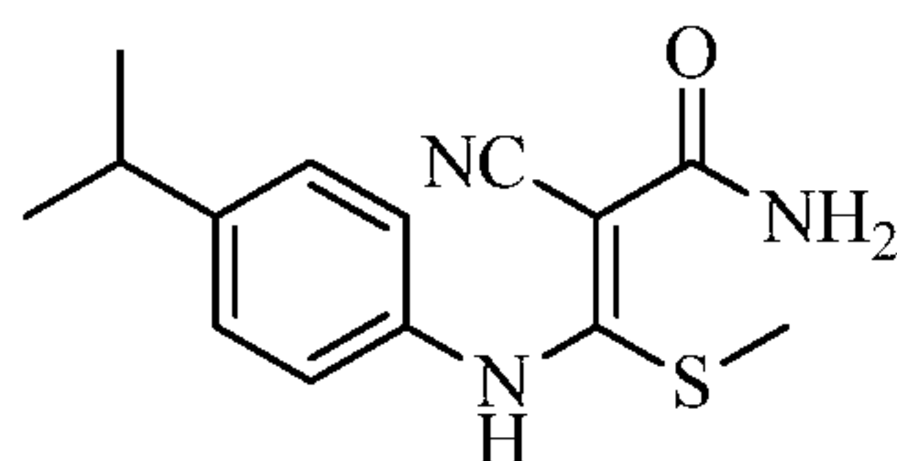
2-cyano-3-((4-isopropylphenyl)amino)-3-(methylthio)acrylamide
