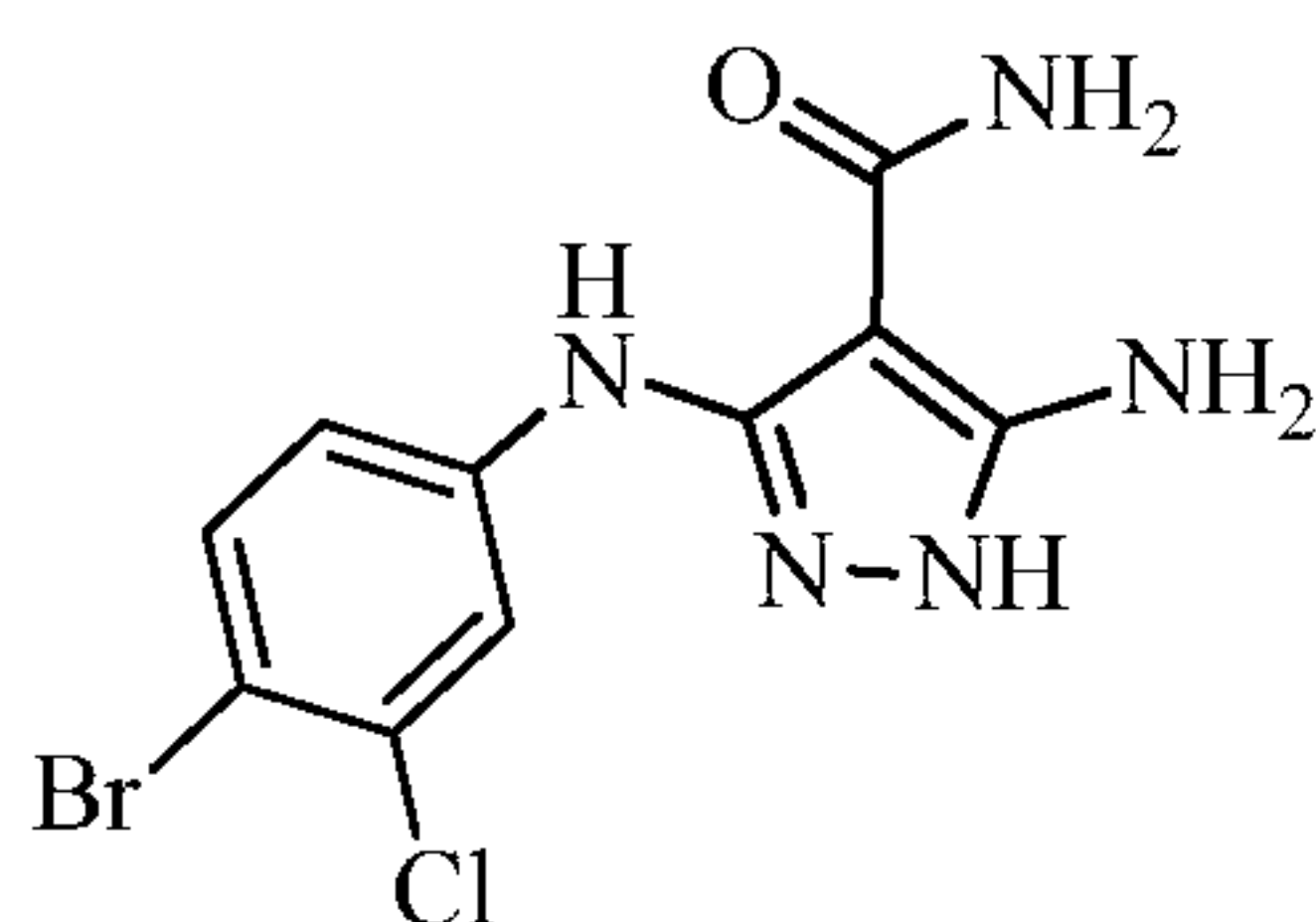
5-amino-3-((4-bromo-3-chlorophenyl)amino)-1 H -pyrazole-4-carboxamide
