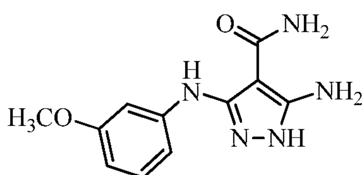
5-amino-3-((3-methoxyphenyl)amino)-1 H -pyrazole-4-carboxamide
