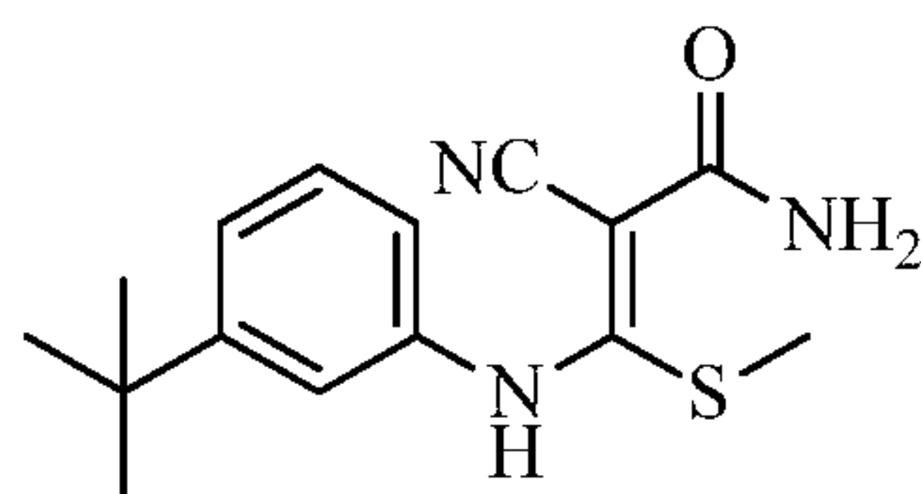
3-((3-(tert-butyl)phenyl)amino)-2-cyano-3-(methylthio)acrylamide
