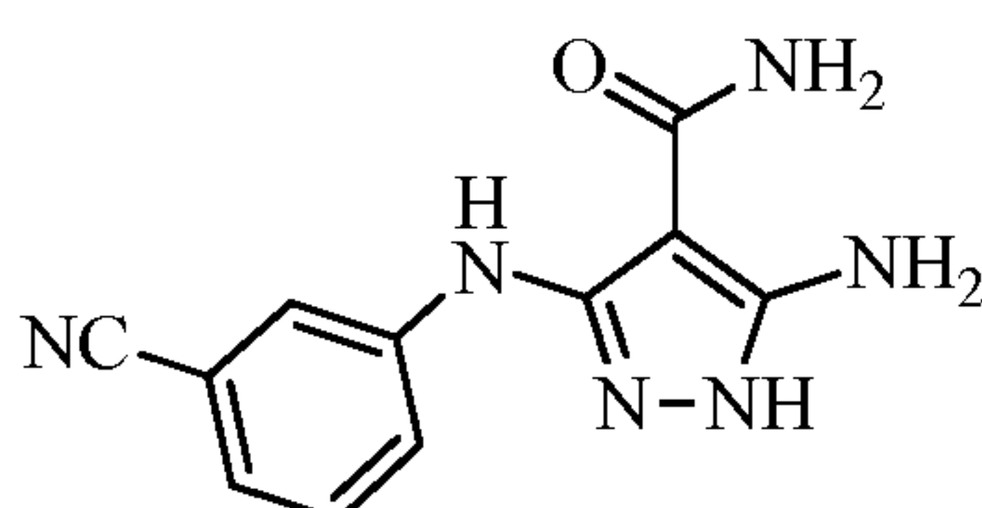
5-amino-3-((3-cyanophenyl)amino)-1 H -pyrazole-4-carboxamide
