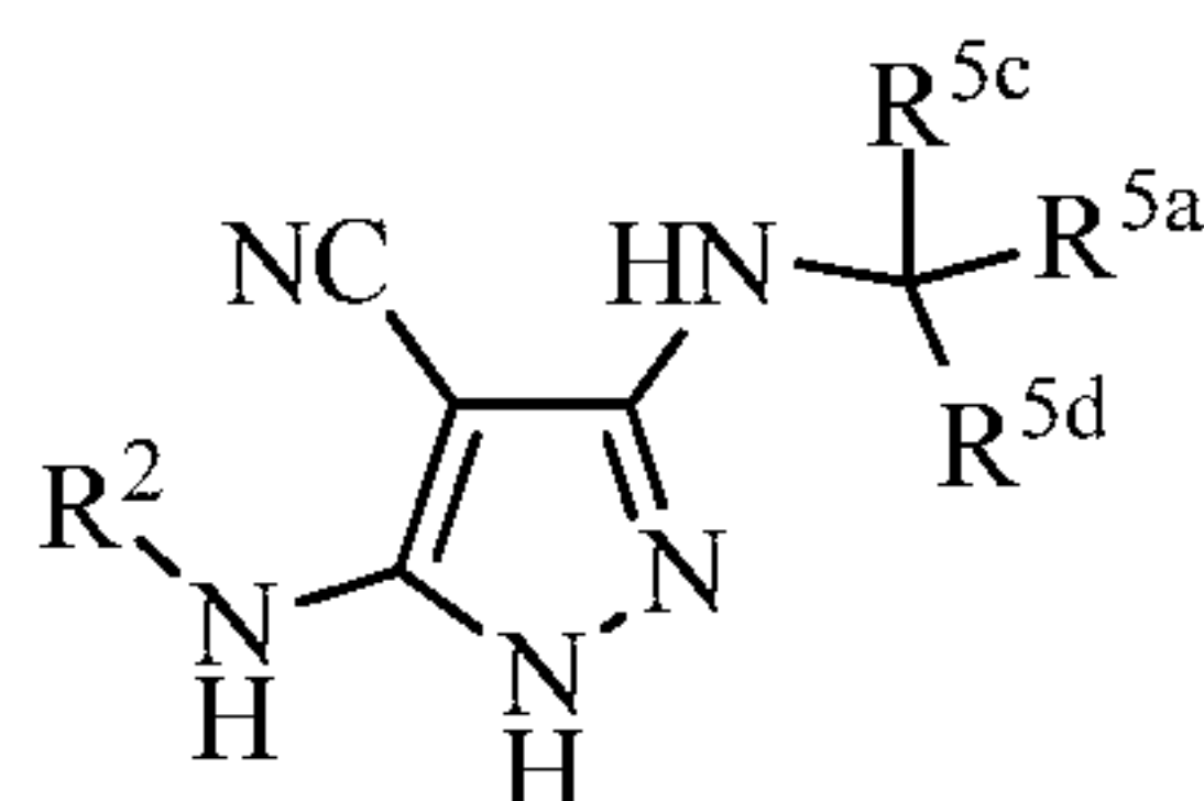
(XIV-c)
