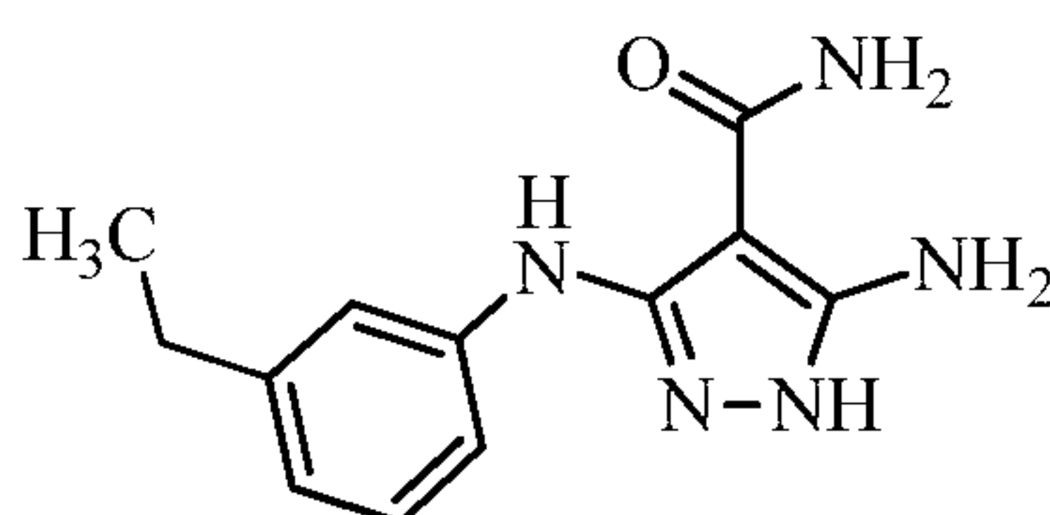
5-amino-3-((3-ethylphenyl)amino)-1 H -pyrazole-4-carboxamide
