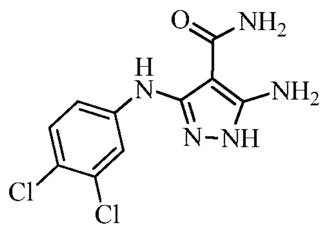
5-amino-3-((3,4-dichlorophenyl)amino)-1 H -pyrazole-4-carboxamide
