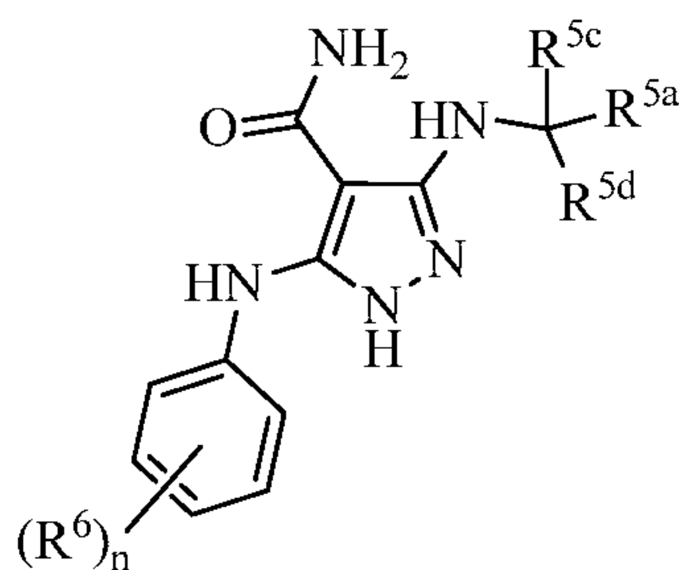
(XVII-c)
