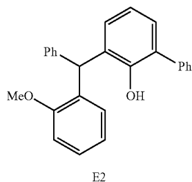
(2-(Benzyloxy)biphenyl-3-yl)(2-methoxyphenyl) methanol (21)
