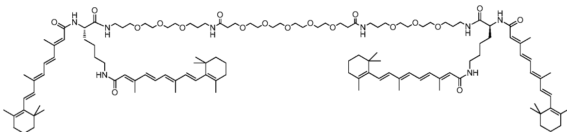
DiVA-PEG-DiVA
