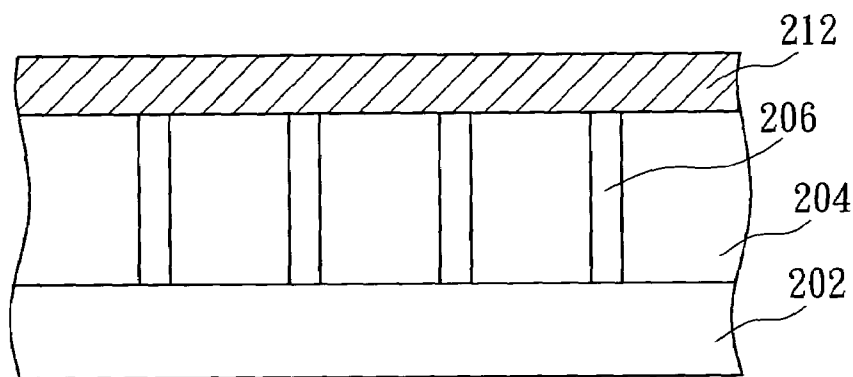
FIG. 2B(PRIOR ART)
