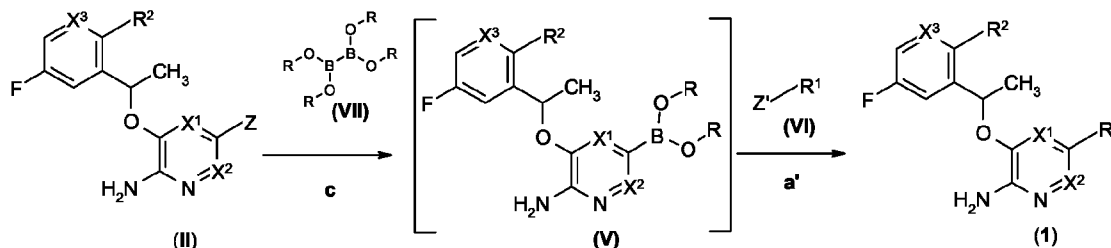
Scheme 1.4
