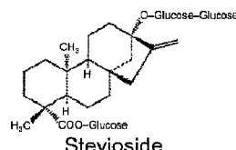
Stevioside
