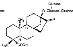
Rebaudioside B
