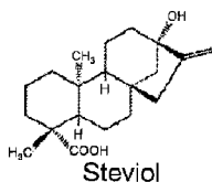
Steviol
