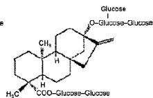
Rebaudioside D
