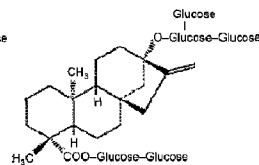
Rebaudioside D
