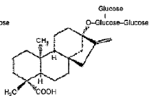
Rebaudioside B
