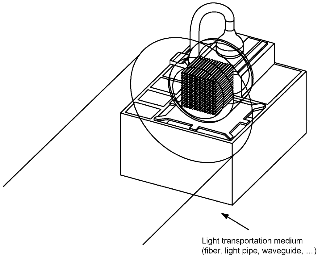
FIG. 22: Array or Module Configuration
