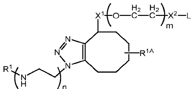
Formula IE-14.
