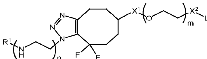
Formula IE-6,
