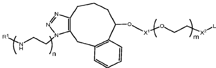
Formula II-4,
