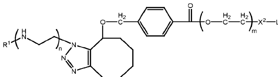
Formula IE-13b,
