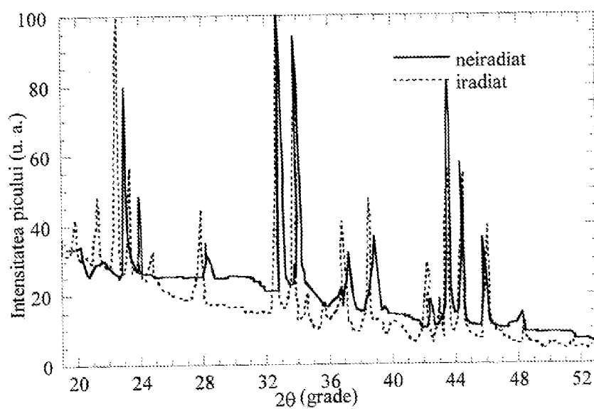
Fig. 3. Difractograma razelor X pentru \text{LaCoO}_3 ( \text{La}_2\text{O}_3 \cdot \text{Co}_2\text{O}_3 ) înainte și după iradiere
