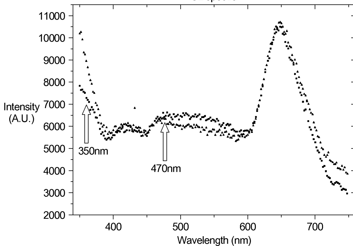
FIG. 6 CL spectra
