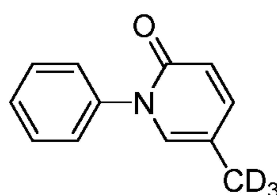
d 3 -pirfenidone.
