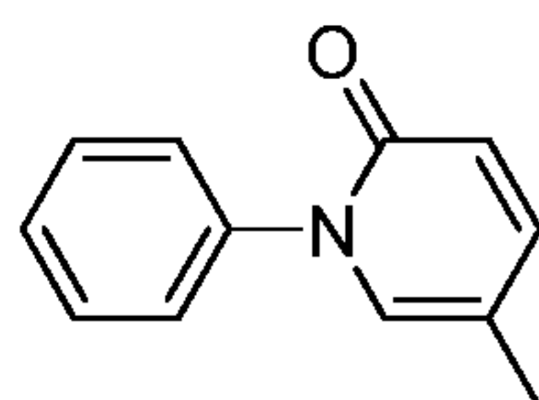
Pirfenidone
