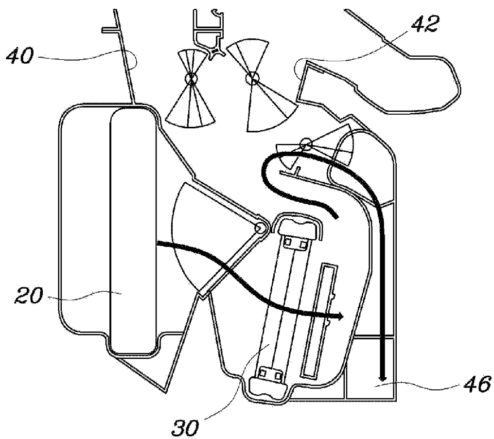
FIG. 7B(Prior Art )
