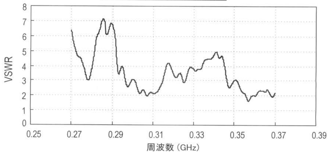
VSWR測定結果 (312MHz)
