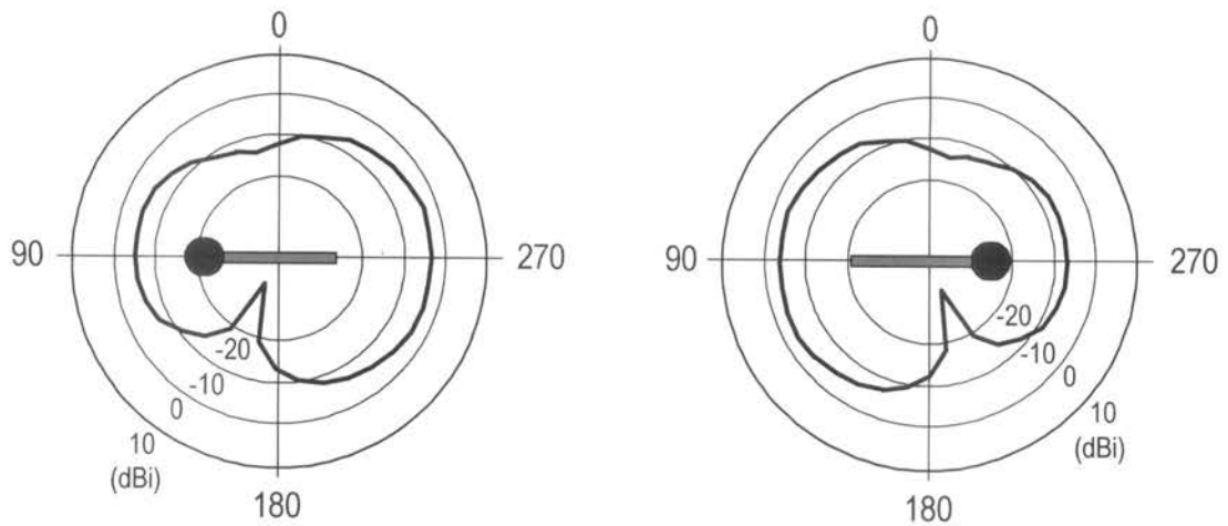
アンテナの指向性測定結果 (312MHz)
