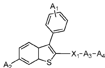
(I-iv)
