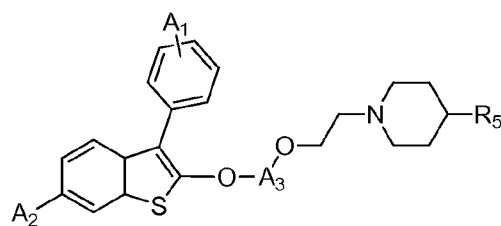
(Ia-iv)
