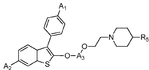
(Ia-vi)
