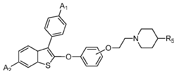
(Ib-vi)
