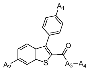
(Ic-vi)
