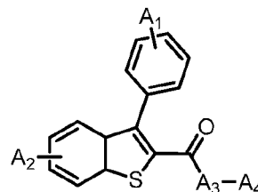
(II-ii)
