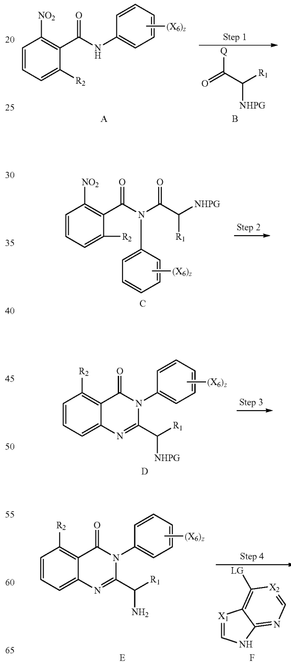
Scheme 1A
