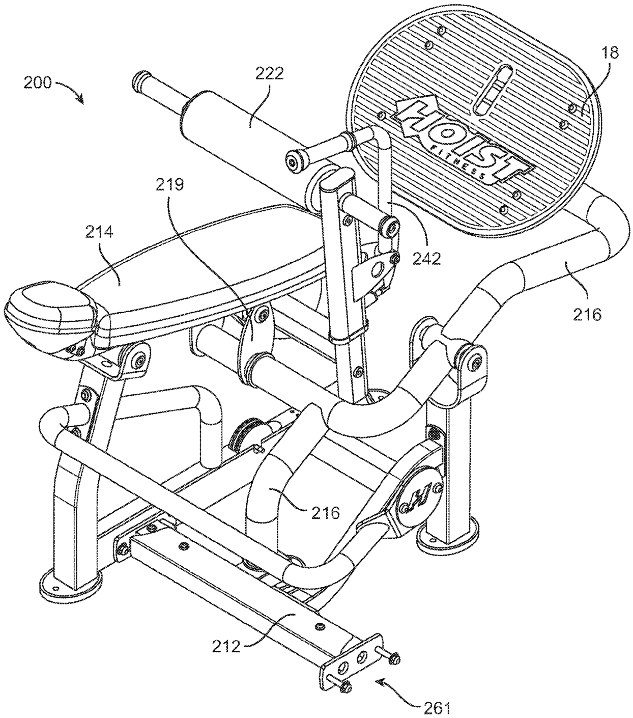
FIG. 21
