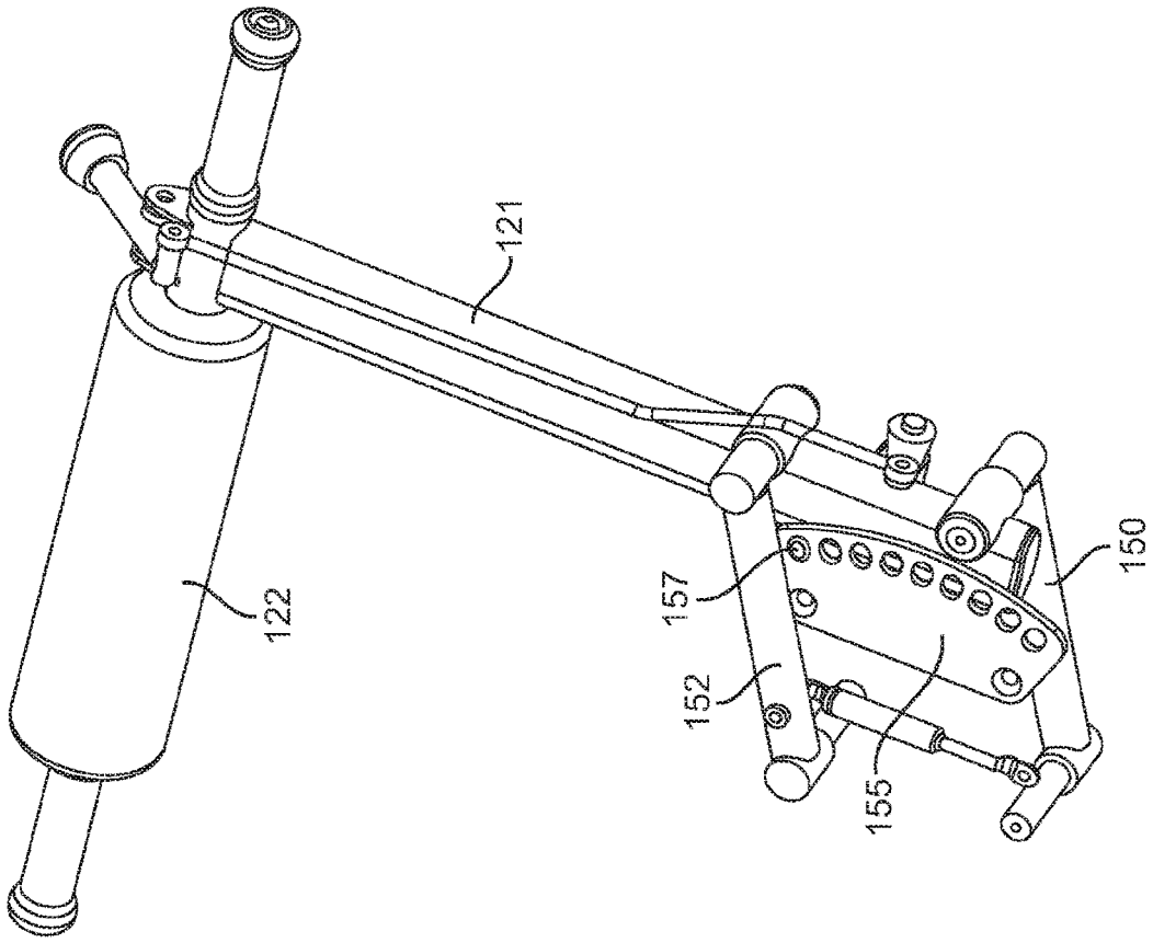
FIG. 16B
