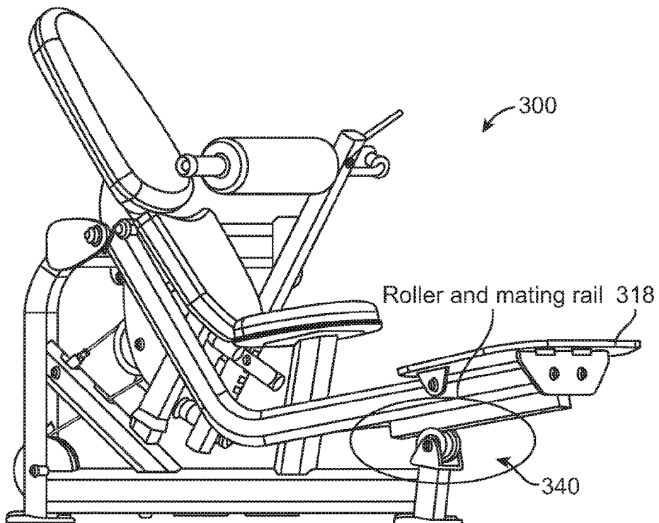
FIG. 24B
