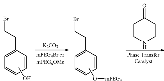
Scheme 11-A
