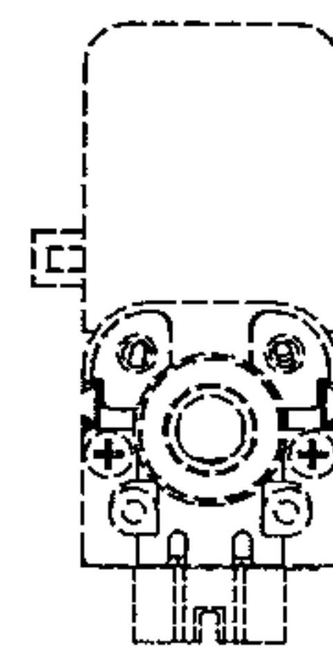
【右側視圖】
