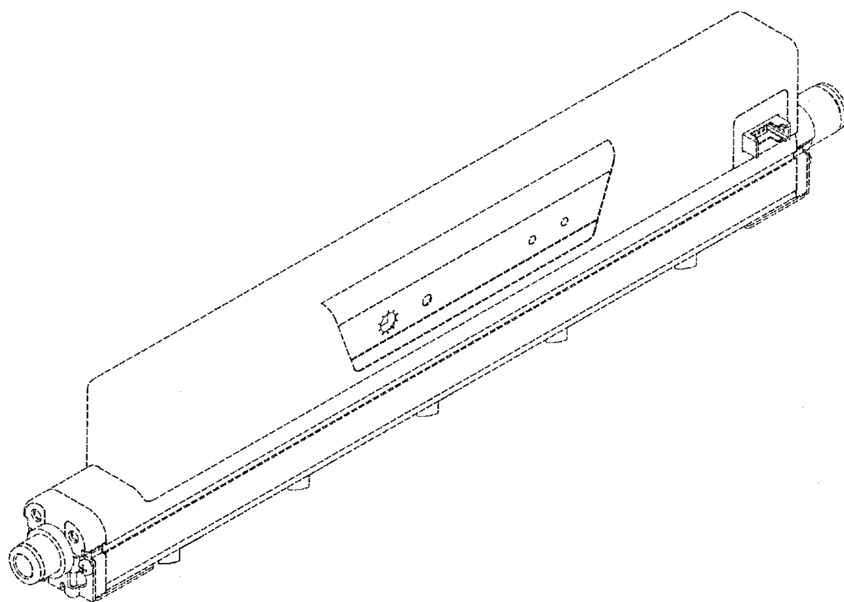
【立體圖1】
