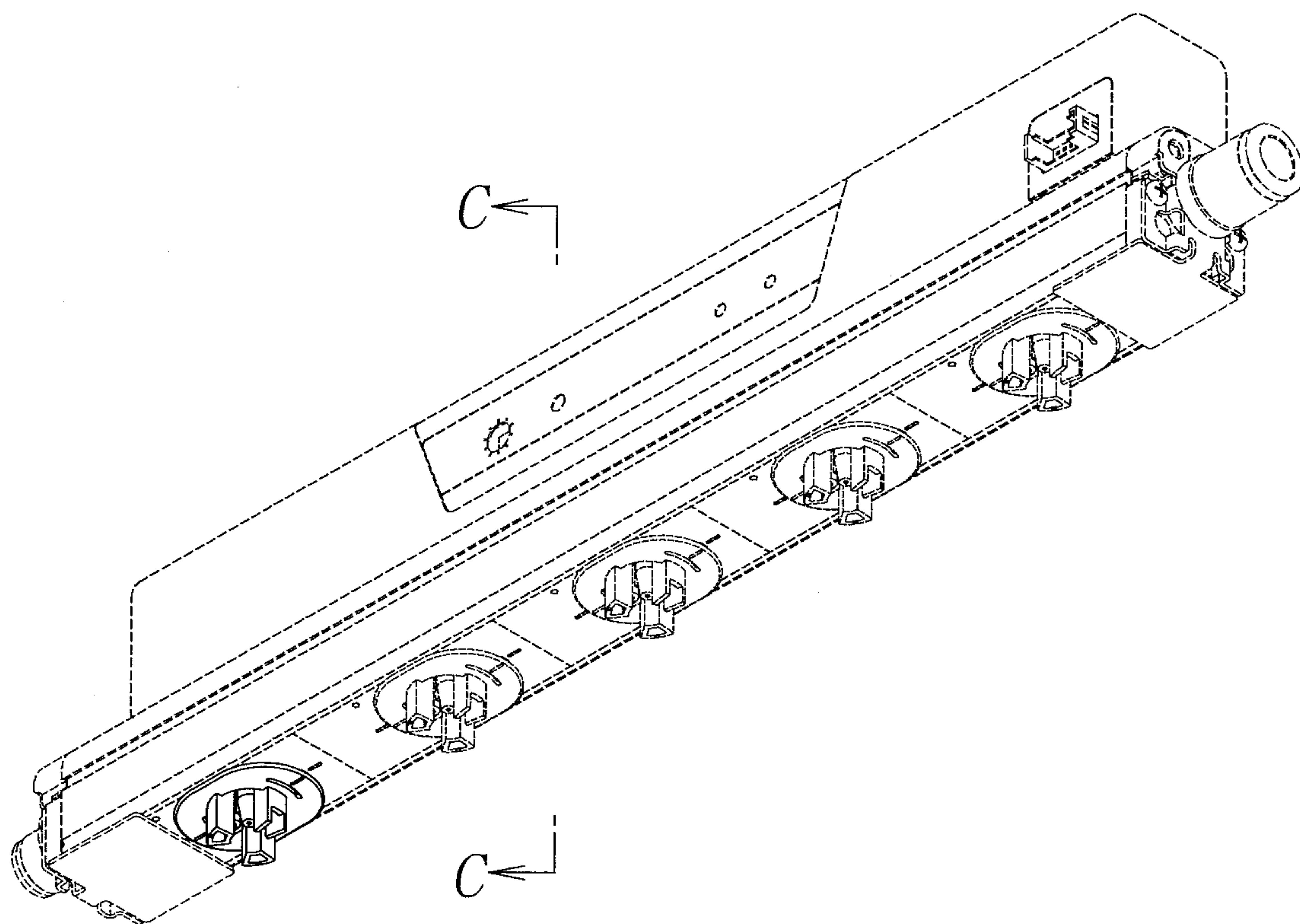
【立體圖 2】
