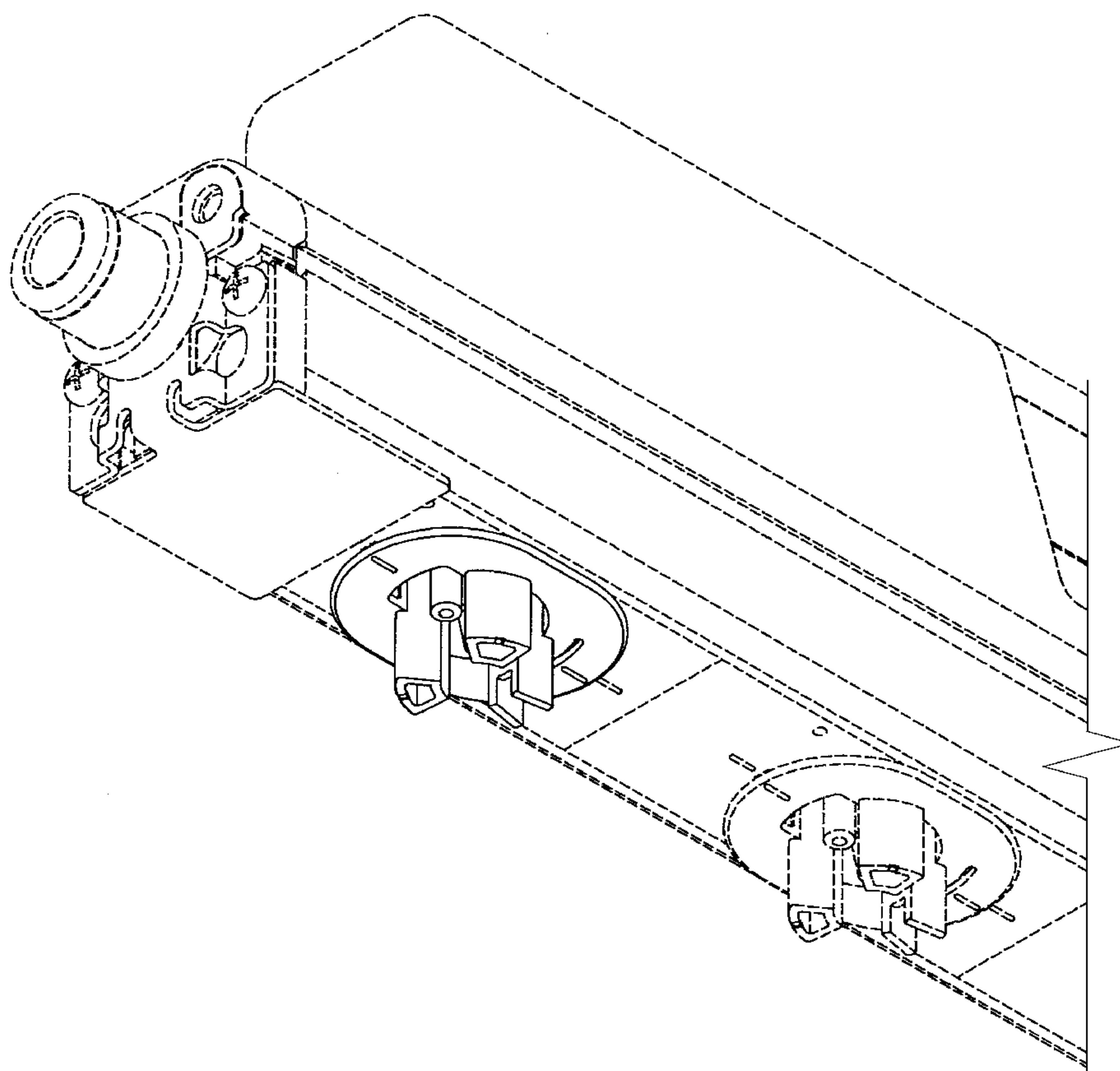
【D-D部分放大圖】
