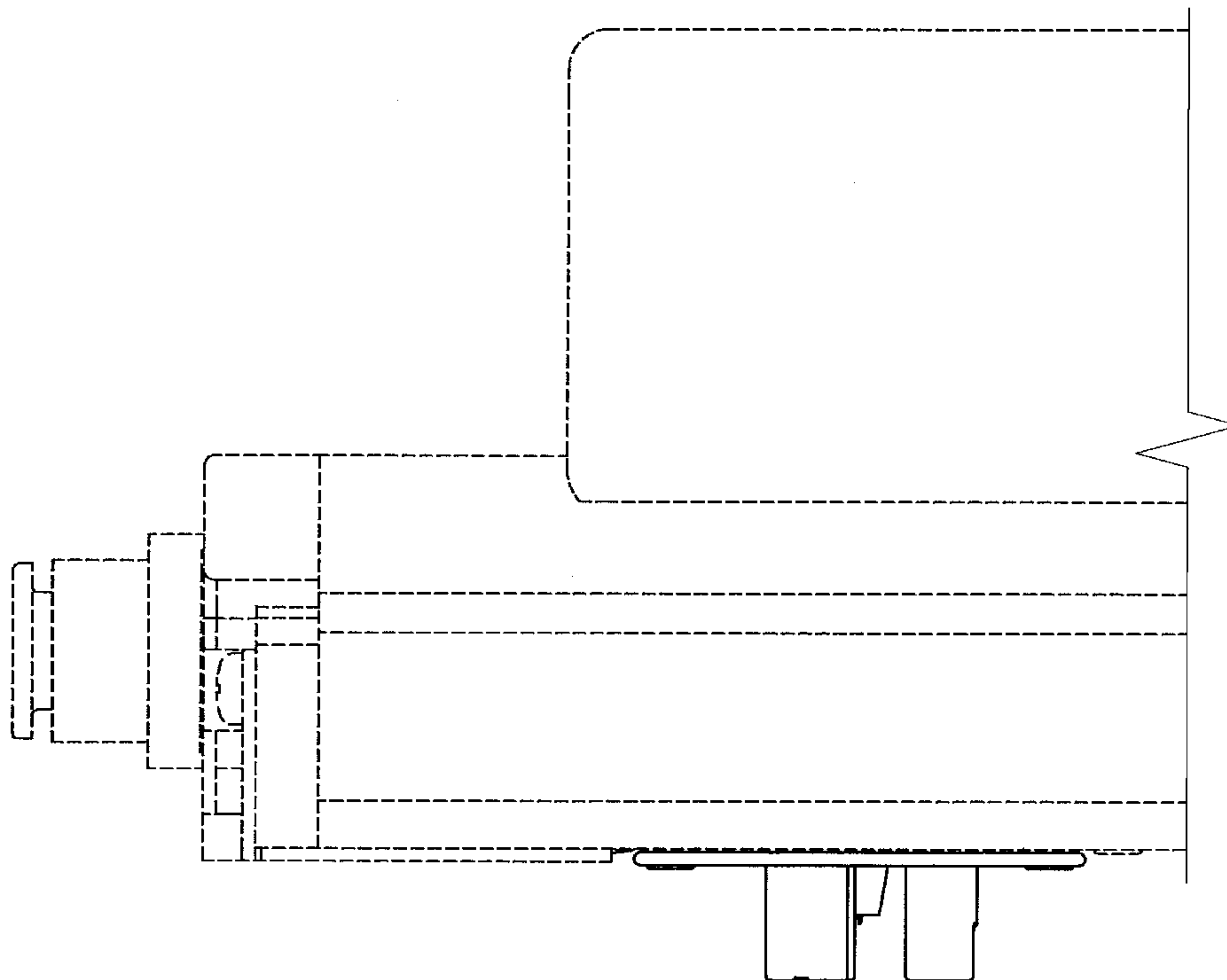
【A-A部分放大圖】
