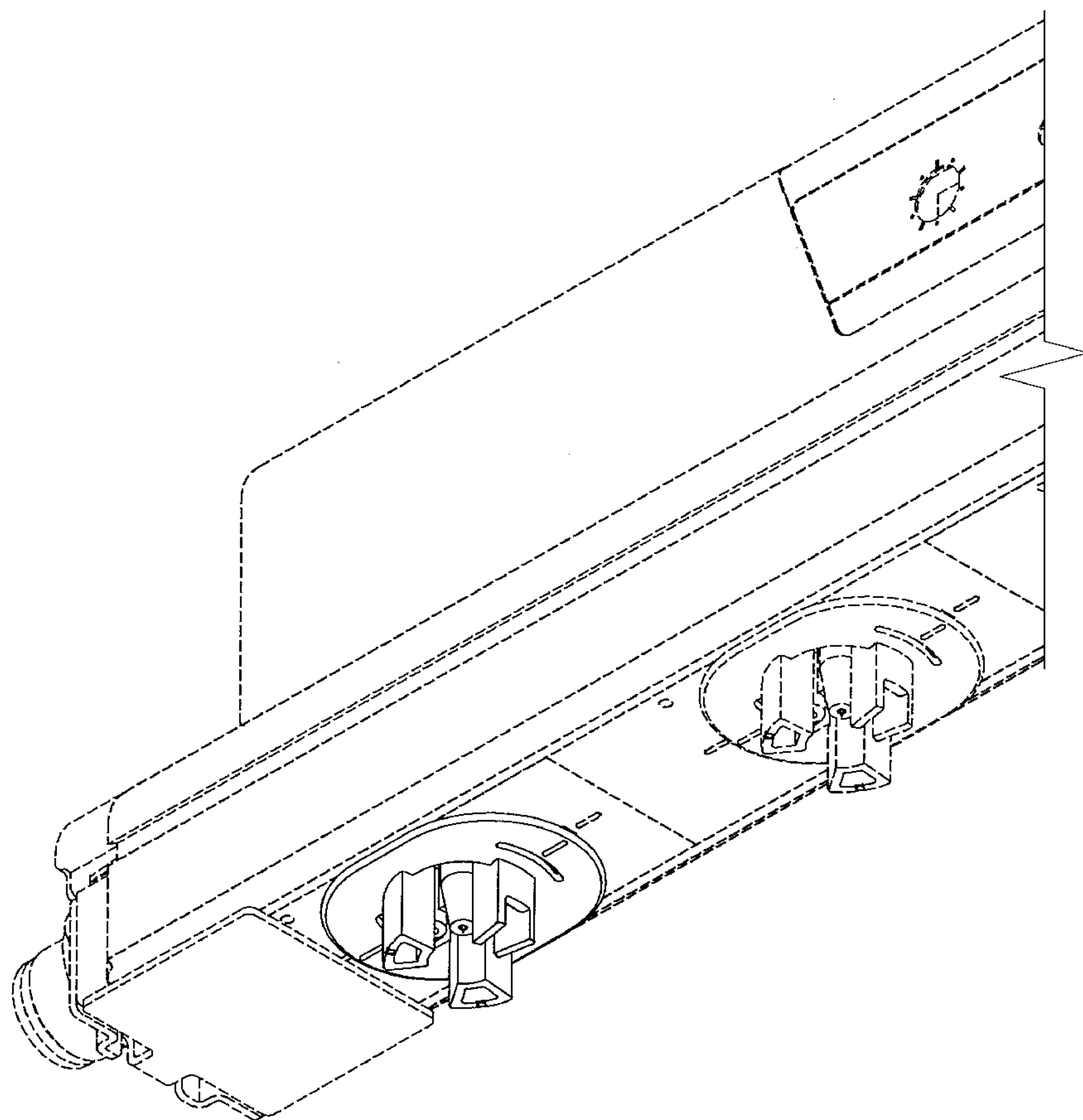
【C-C部分放大圖】
