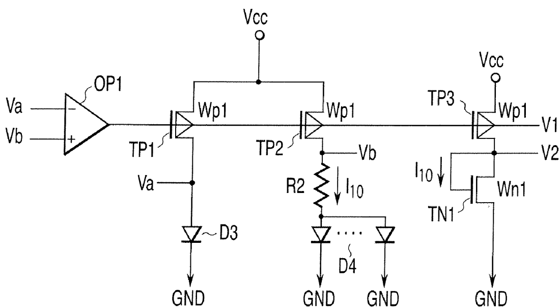
FIG. 8A
