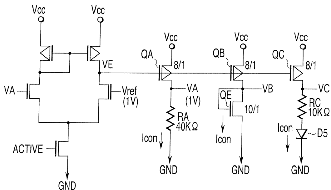
FIG. 11A
