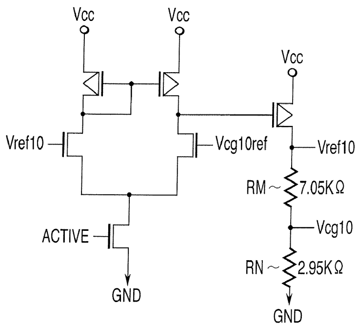
FIG. 14B
