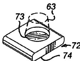
FIG. 31A
