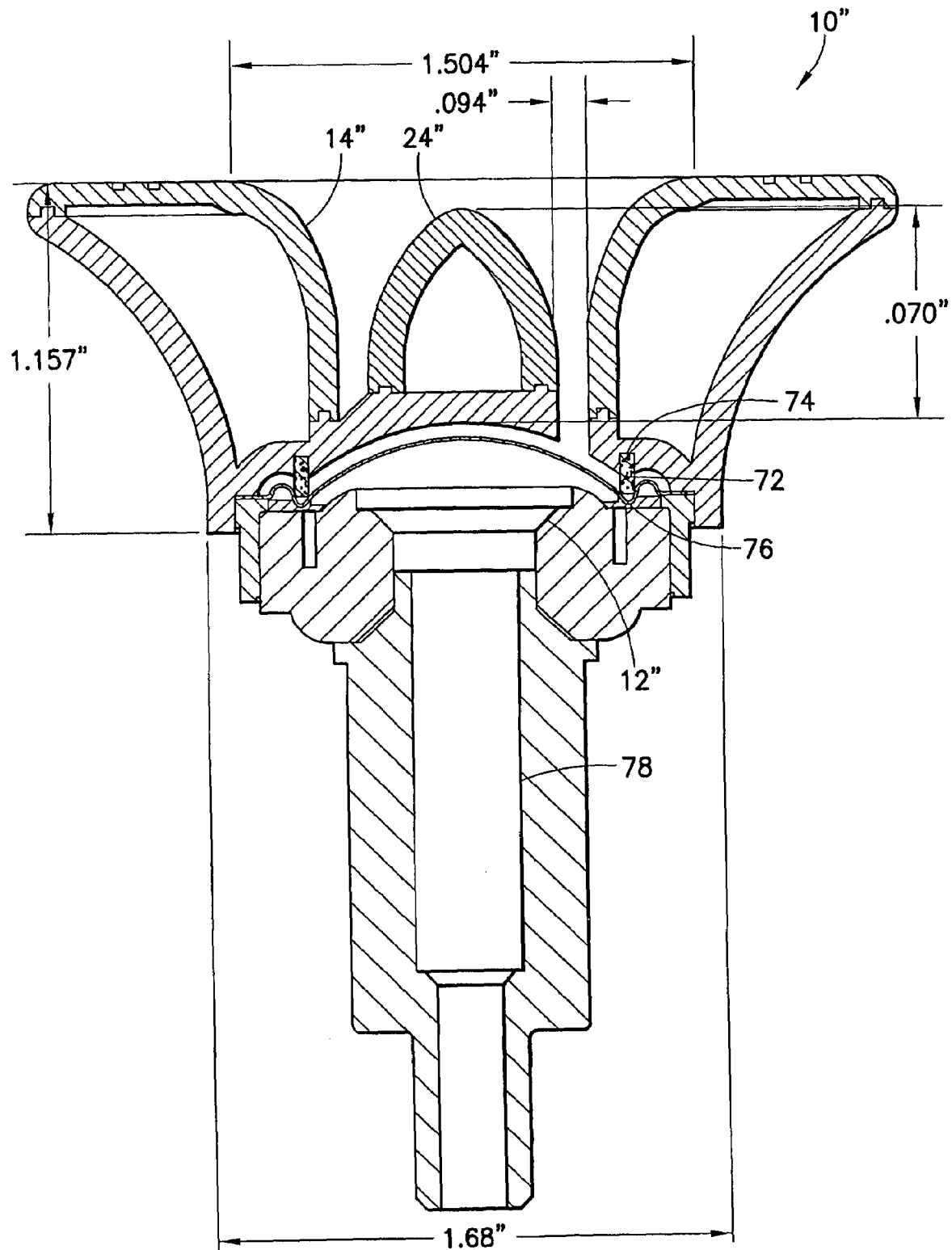
FIG.7B
