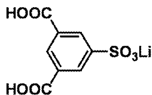
lithium 3,5-dicarboxybenzenesulfonate
