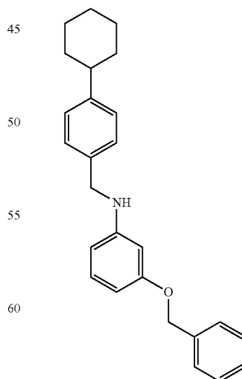
3-(benzyloxy)-N-(4-cyclohexylbenzyl)aniline
