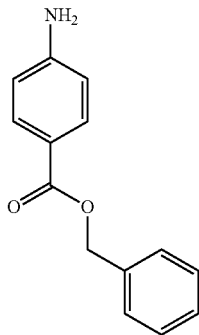
benzyl 4-aminobenzoate
