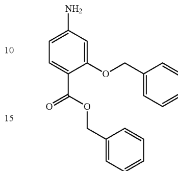
benzyl 4-amino-2-(benzyloxy)benzoate
