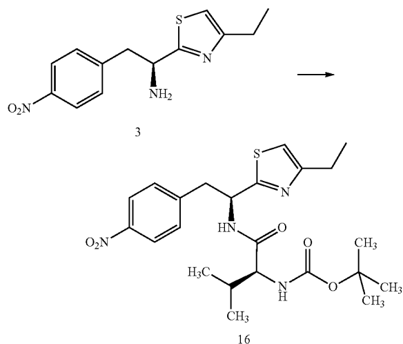
Scheme VI
