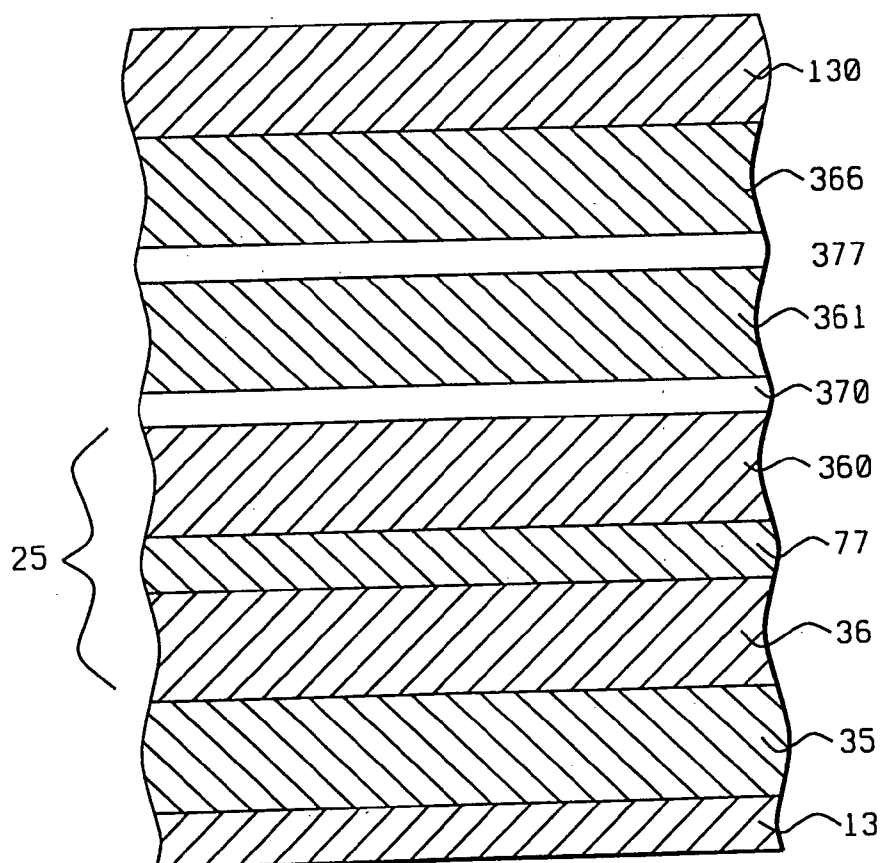
FIG. 4d
