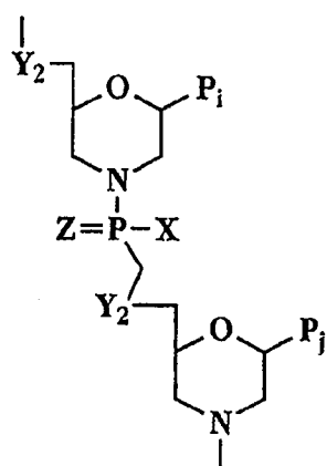
Fig. 2C-C
