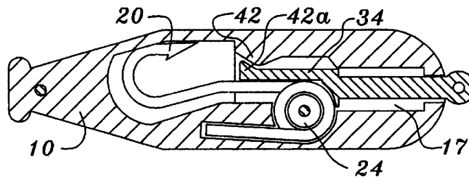
Fig. 3 VIEW A-A
