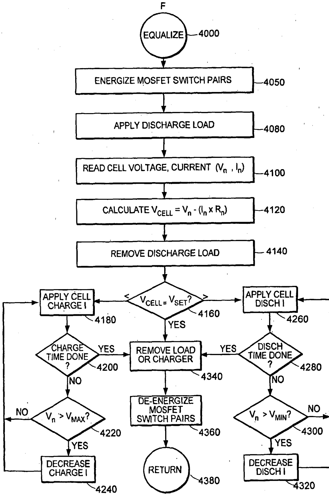
G FIG. 7D
