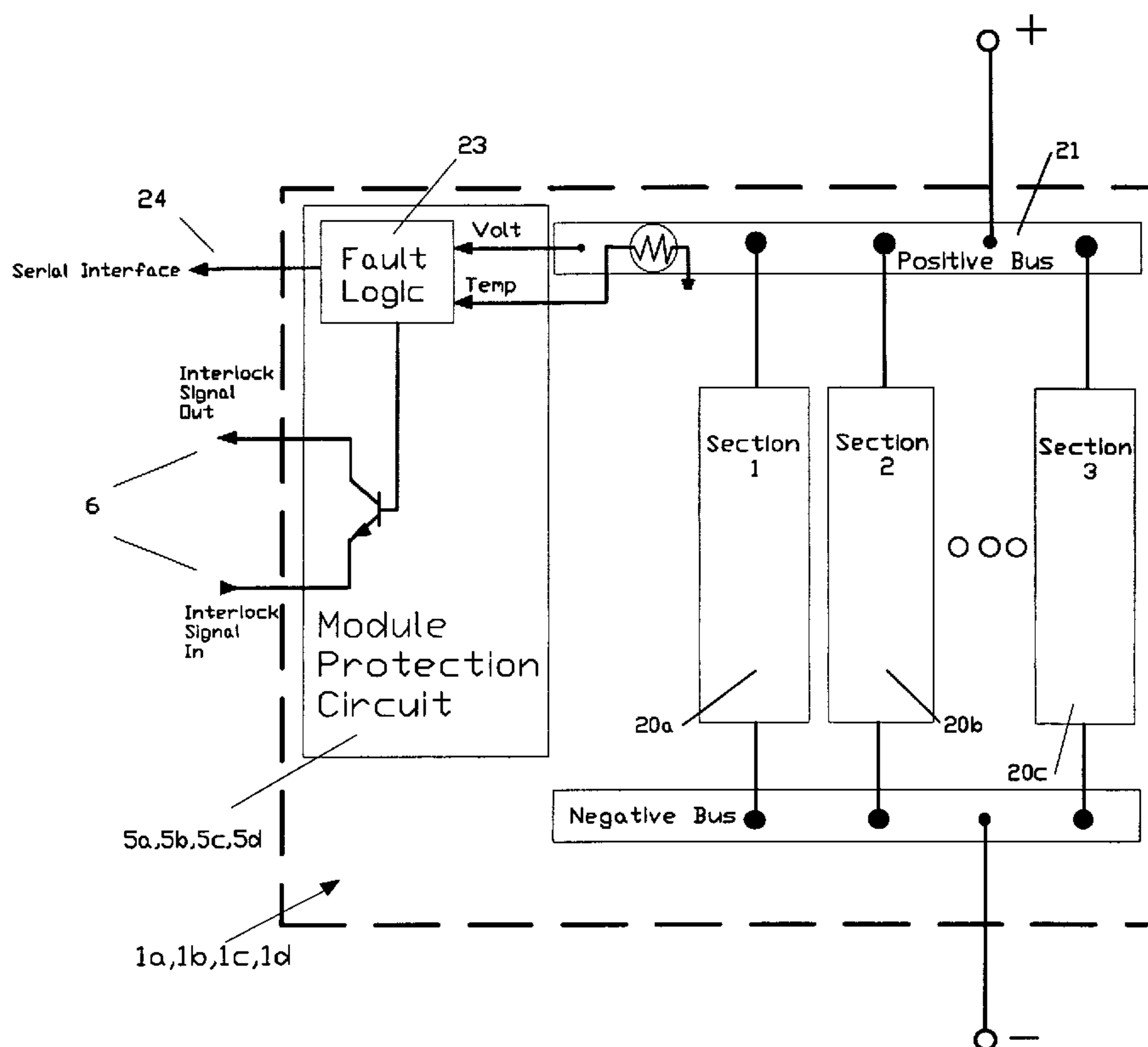
Battery Module
