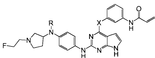
I-30 (X=O, NH, CH 2 , CF 2 ; R=H, CH 3 )
